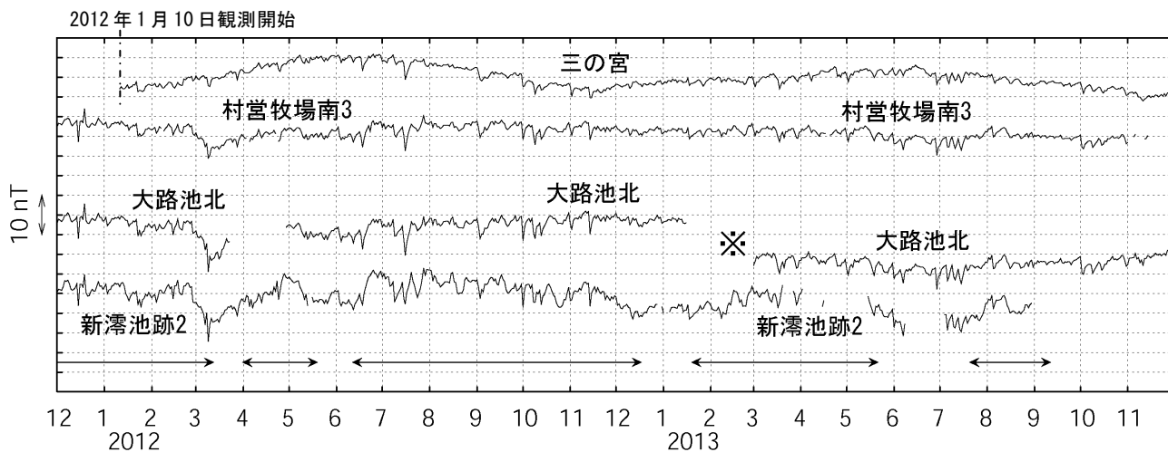
図4 三宅島 全磁力連続観測による全磁力値の変化 (2011 年 12 月～2013 年 11 月) 基準点 : 雄山北東
