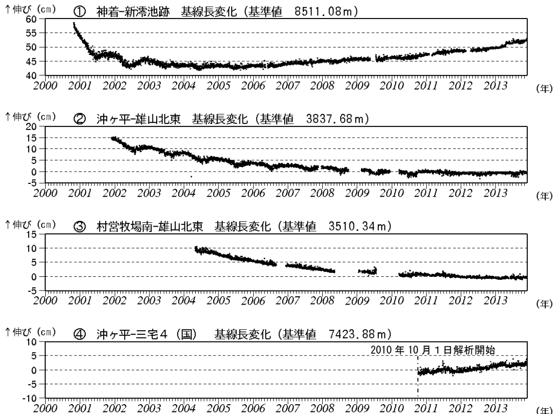
図3 三宅島 GPS 連続観測結果 (2000 年 1 月～2013 年 11 月) (国) : 国土地理院 ・ 基線①～④は図7 (観測点配置図) の①～④にそれぞれ対応します。 ・ グラフの空白部分は欠測を示します。 ・ 2010 年 10 月以降のデータについては、電離層の影響を補正する等、解析方法を改良しています。
