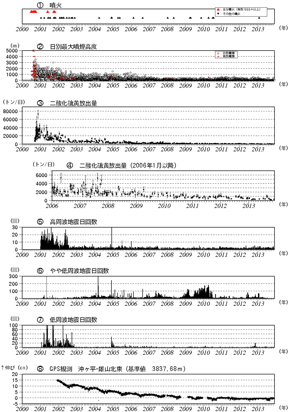
図2 三宅島 最近の火山活動の経過図 (2000年1月～2013年11月)
