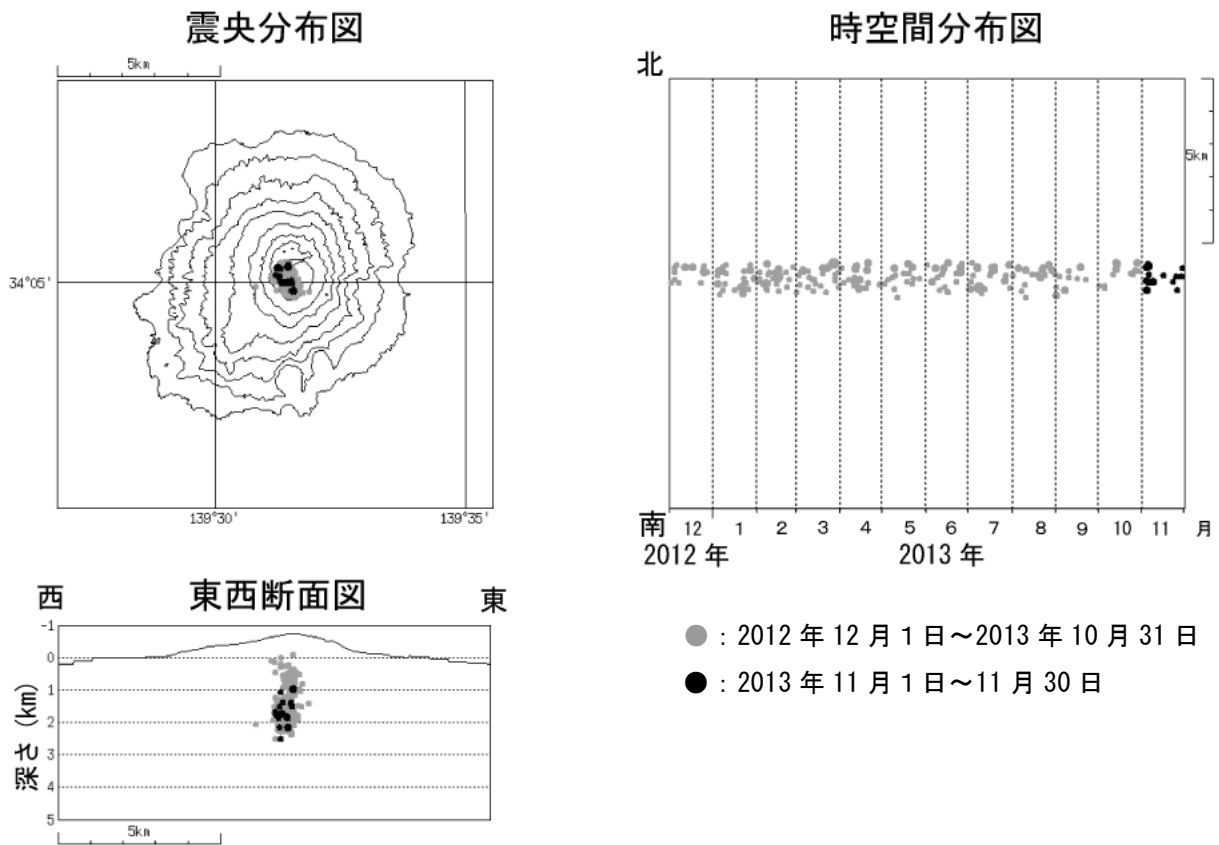
図5 三宅島 震源分布図 (2012 年 12 月 1 日 ~ 2013 年 11 月 30 日)
