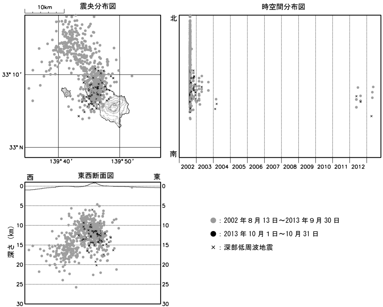
図3 八丈島 震源分布図（2002年8月13日～2013年10月31日） 今期間、八丈島付近に震源が決定された高周波地震及び深部低周波地震はありませんでした。
