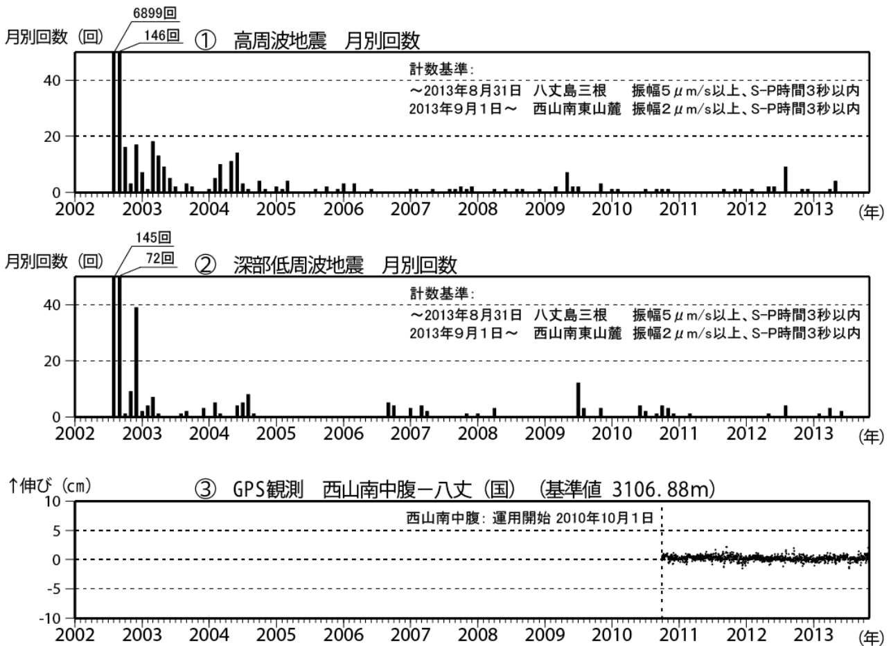
図2 八丈島 火山活動の経過図 (2002年8月13日~2013年10月31日)
