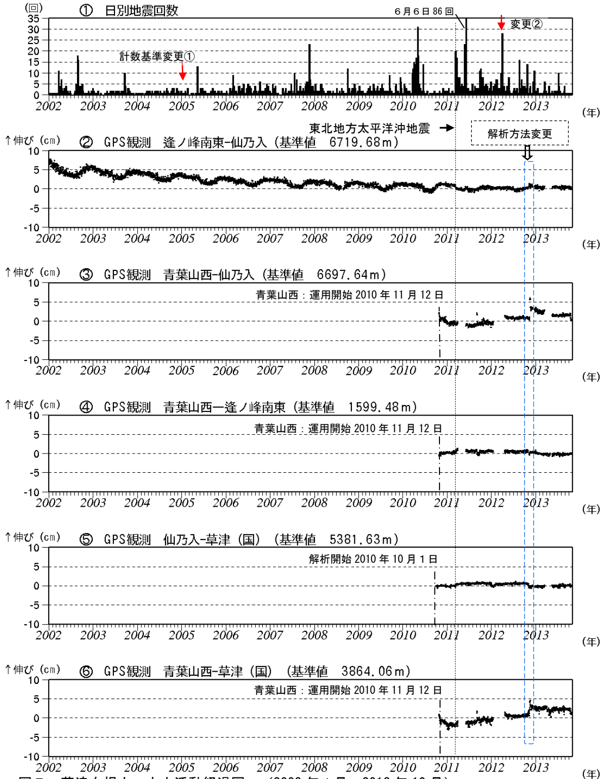
図5 草津白根山 火山活動経過図 (2002年1月～2013年10月)
