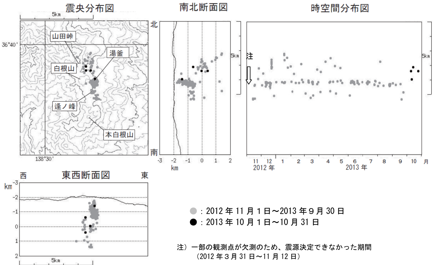
図4 草津白根山 震源分布図（2012年11月1日～2013年10月31日）
