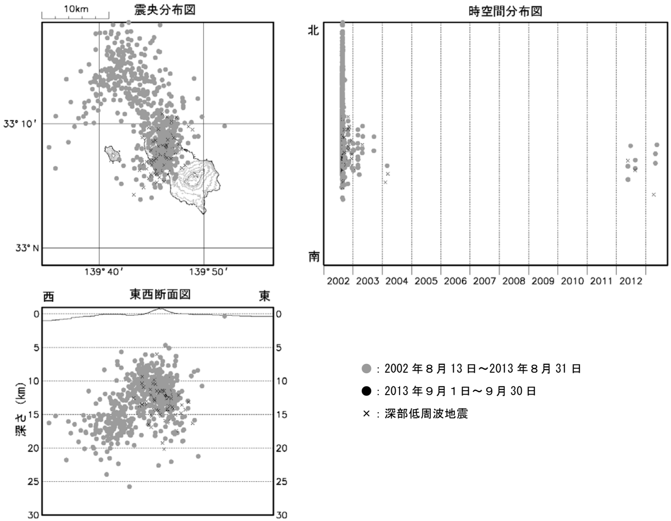
図3 八丈島 震源分布図 (2002年8月13日~2013年9月30日) 今期間、八丈島付近に震源が決定された高周波地震及び深部低周波地震はありませんでした。
