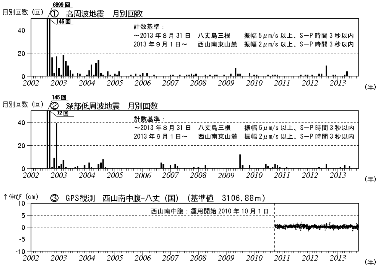
図 2 八丈島 火山活動の経過図 (2002 年 8 月 13 日~2013 年 9 月 30 日)
