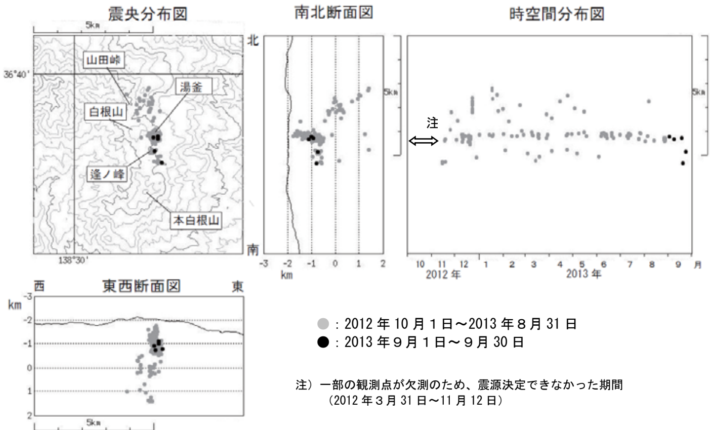
図4 草津白根山 震源分布図（2012年10月1日～2013年9月30日）
