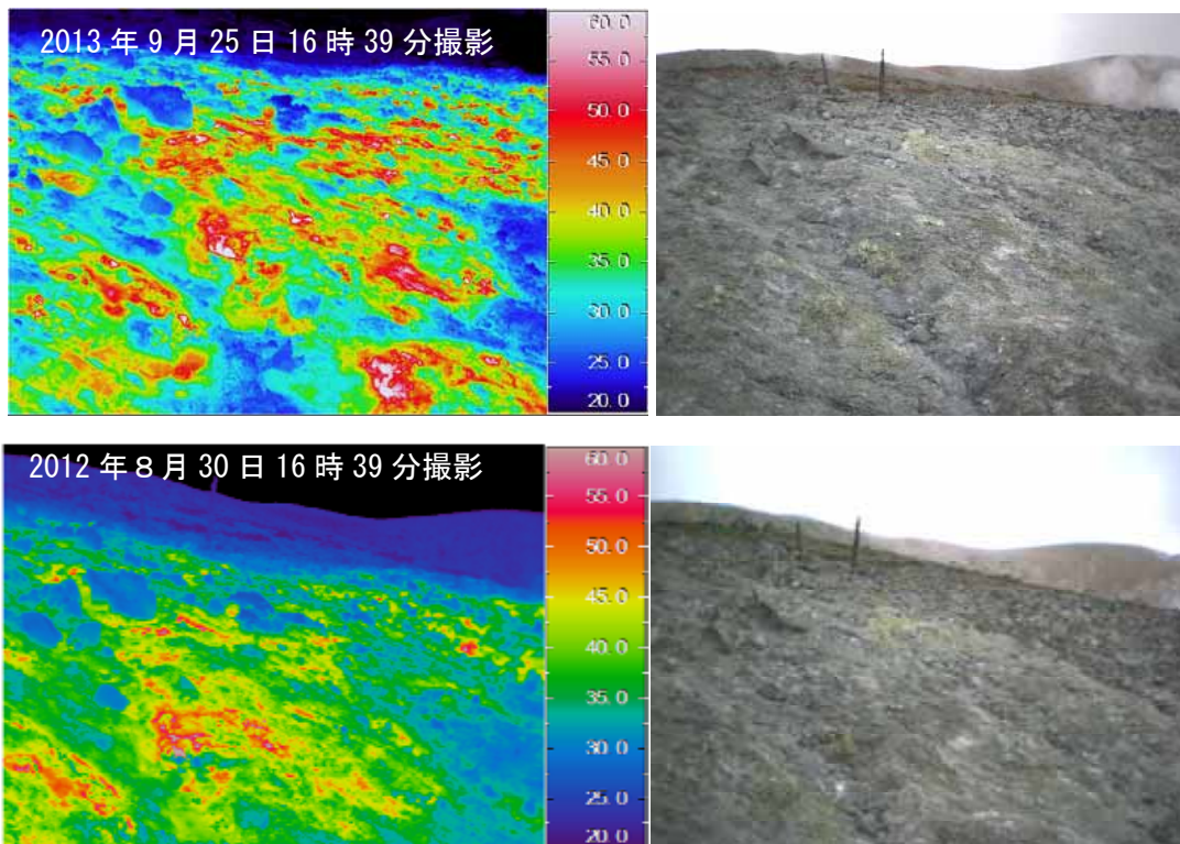
図7 草津白根山 水釜火口北側斜面の状況と地表面温度分布 撮影地点と撮影方向は図7を参照。
