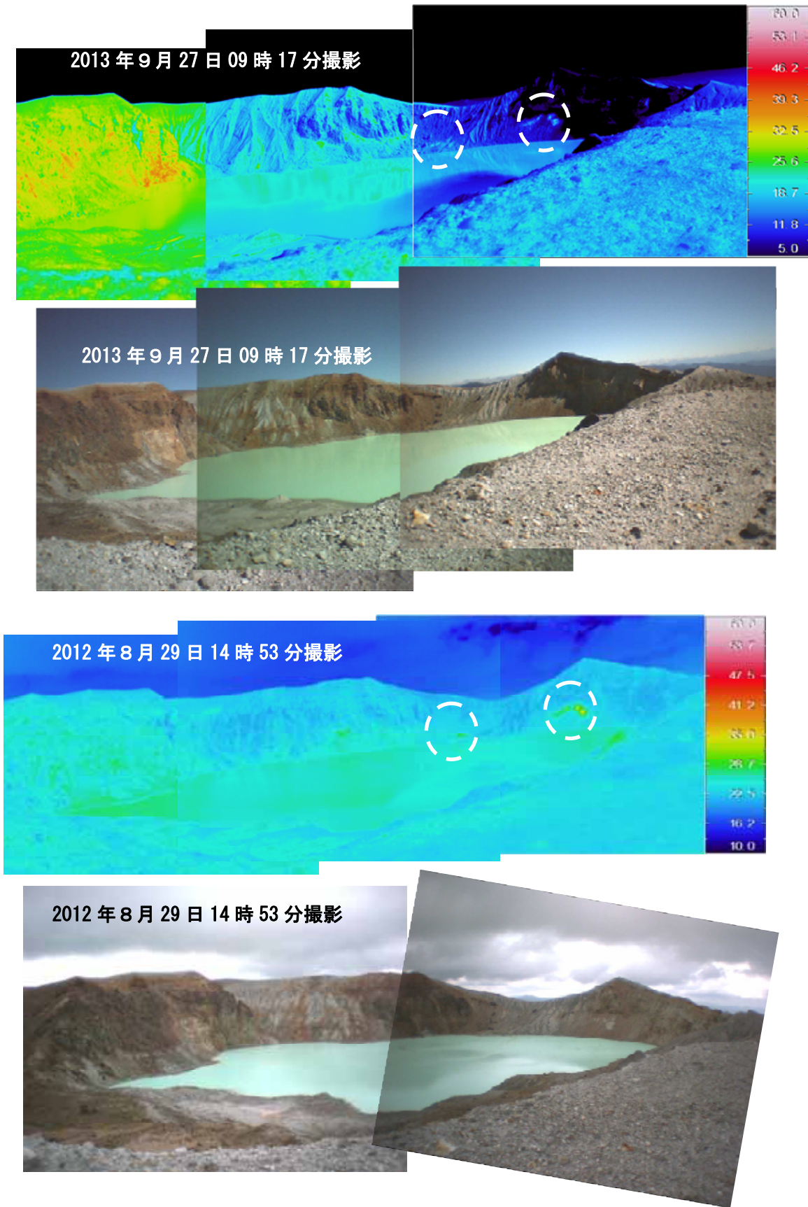
図 8 草津白根山 湯釜の南側から撮影した湯釜火口内北壁の状況と地表面温度分布 撮影地点と撮影方向は図 7 を参照。 湯釜火口内北壁は熱活動の活発な状況が続いており、引き続き高温領域（白破線の円）が認められました。
