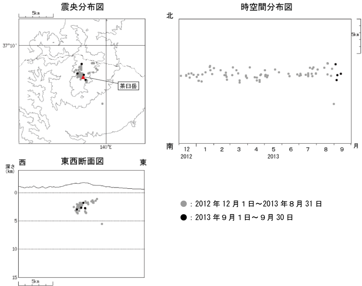
図3 那須岳 那須岳の地震観測点による震源分布図（2012 年 12 月 1 日～2013 年 9 月 30 日） 震源は主に山頂直下のごく浅い所に分布しました。
