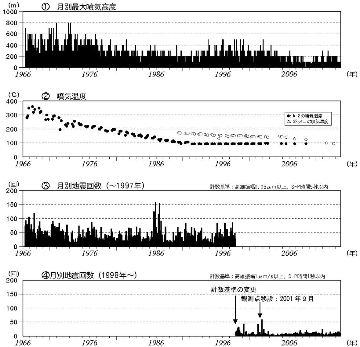
図2 那須岳 火山活動経過図 (1966年1月~2013年9月)
