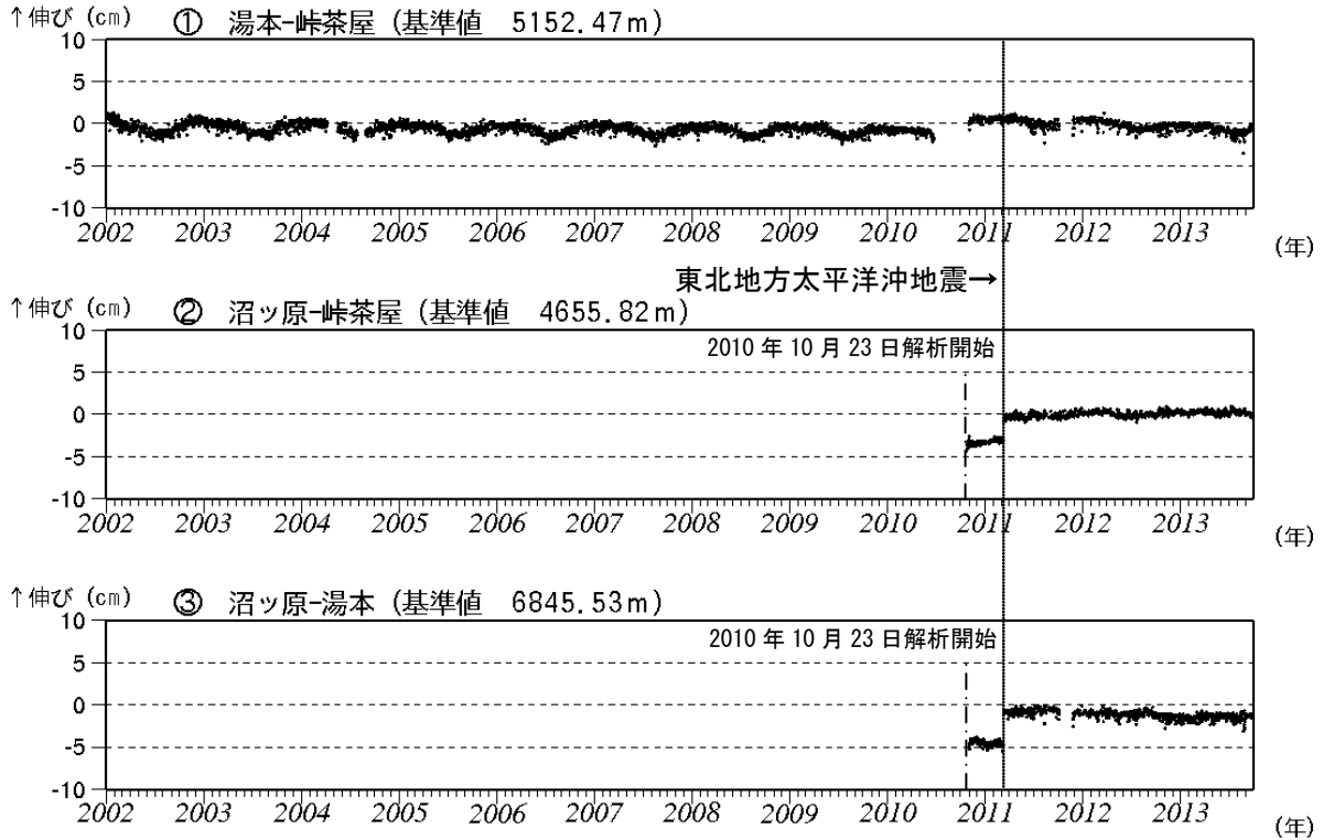
図4 那須岳 GPS 連続観測による基線長変化 (2002 年 1 月～2013 年 9 月) 2010 年 10 月以降のデータについては、電離層の影響を補正する等、解析方法を改良しています。 基線長変化にみられる冬季の伸びと夏季の縮みの傾向は季節変動による変化です。 2011 年 3 月 11 日に発生した東北地方太平洋沖地震の影響により、データに飛びがみられます。 ①～③は図5のGPS基線①～③に対応しています。グラフの空白部分は欠測を示します。
