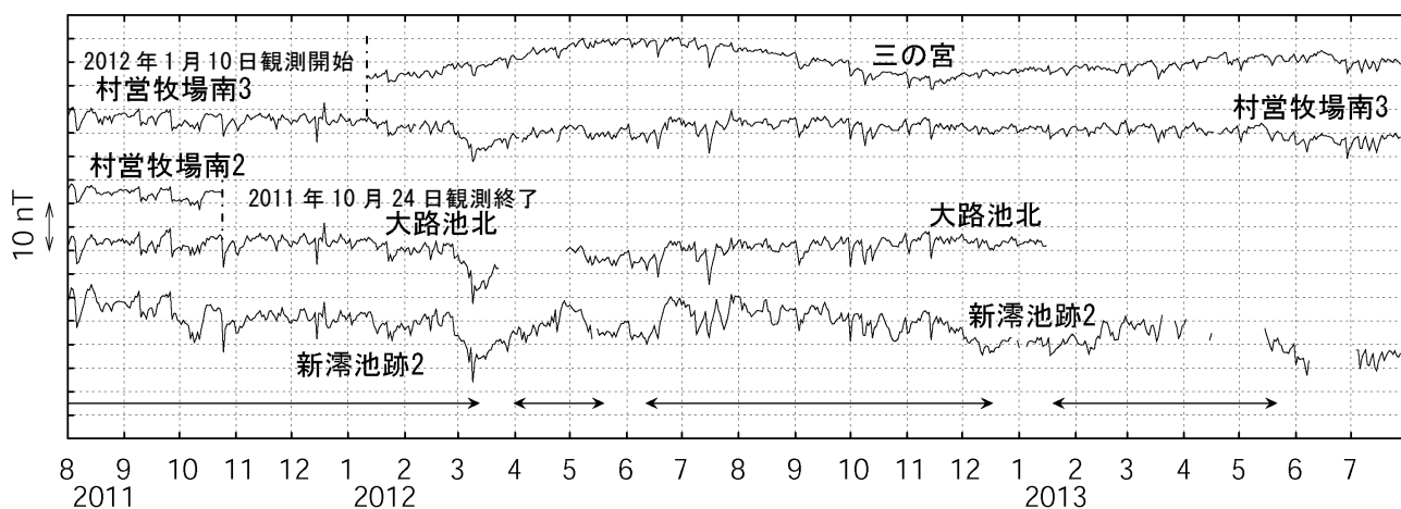
図4 三宅島 全磁力連続観測による全磁力値の変化（2011年7月～2013年7月） 基準点：雄山北東
