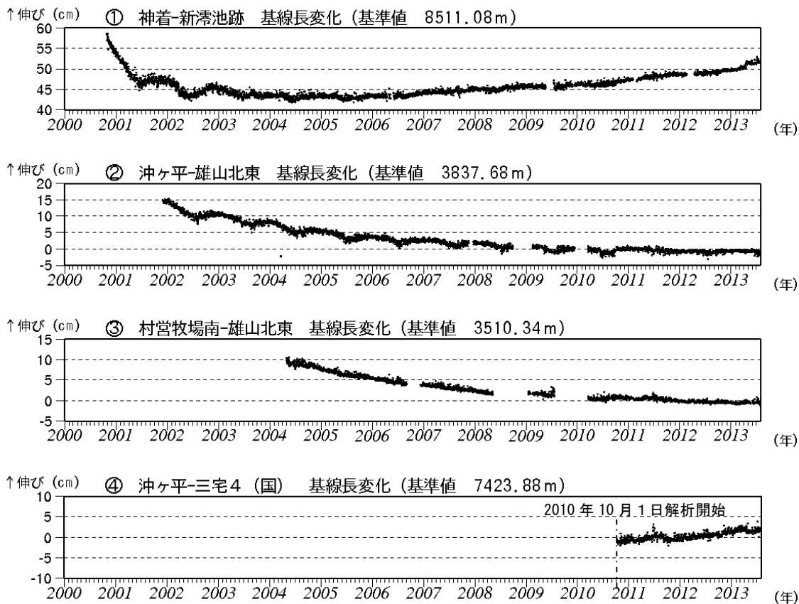
図3 三宅島 GPS 連続観測結果（2000年1月～2013年7月）（国）：国土地理院 ・基線①～④は図7（観測点配置図）の①～④にそれぞれ対応します。 ・グラフの空白部分は欠測を示します。 ・2010年10月以降のデータについては、電離層の影響を補正する等、解析方法を改良しています。
