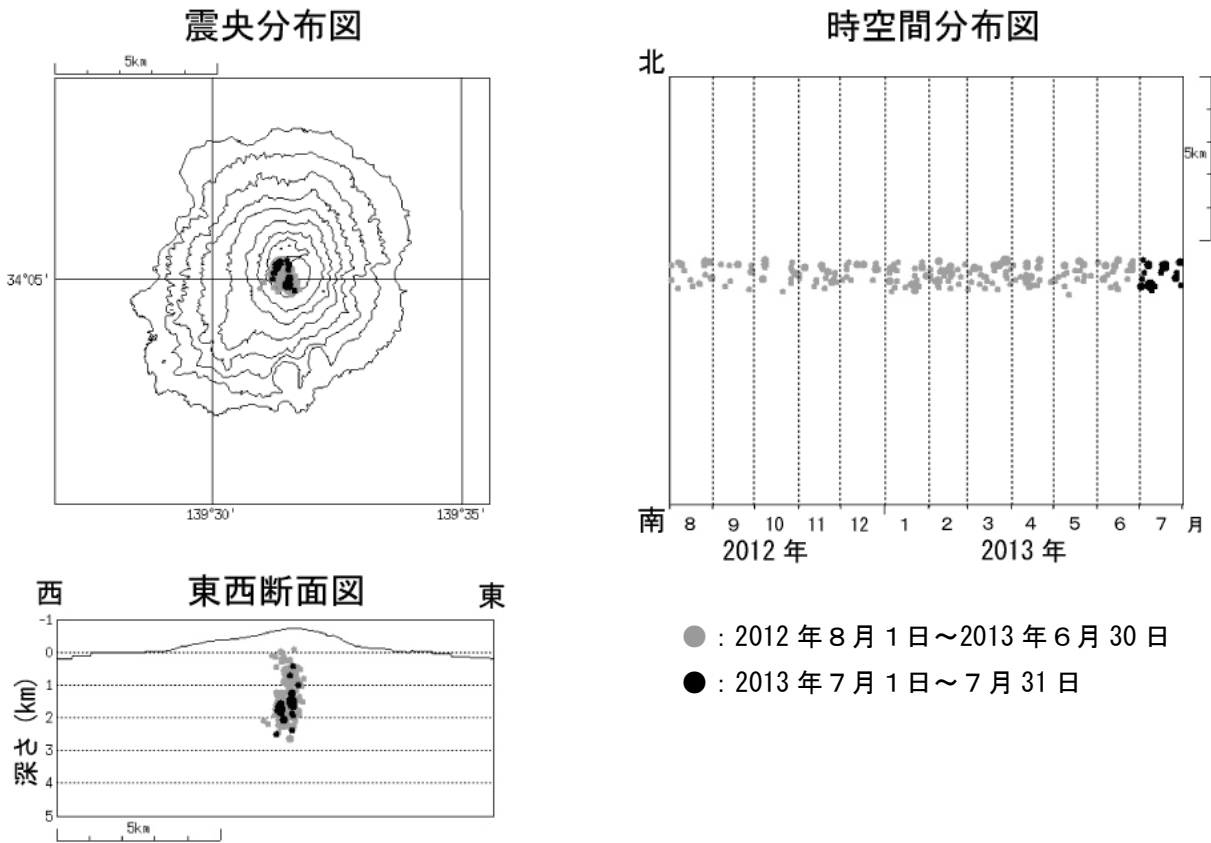
図5 三宅島 震源分布図（2012年8月1日～2013年7月31日）
