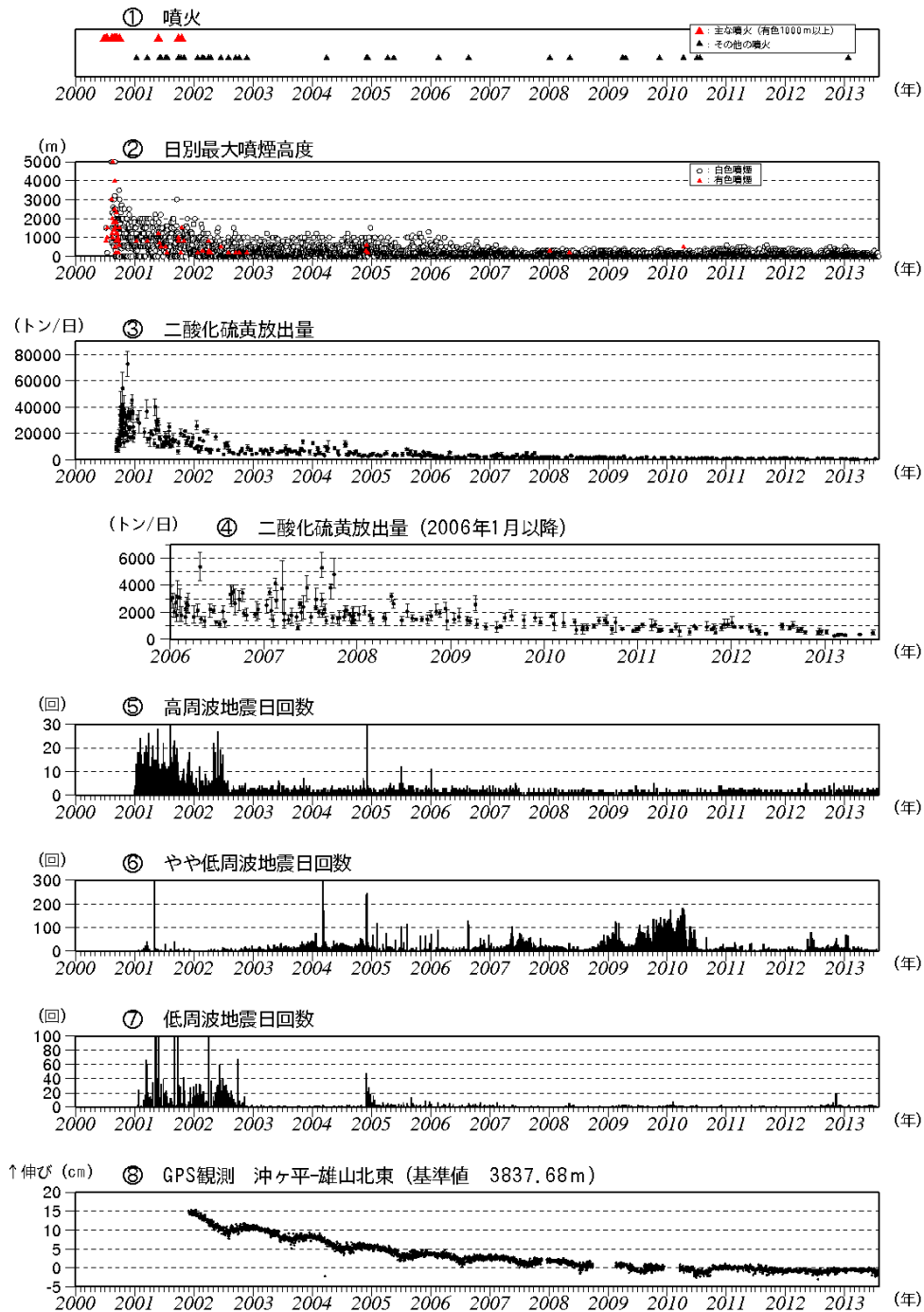
図2 三宅島 最近の火山活動の経過図 (2000年1月~2013年7月)
