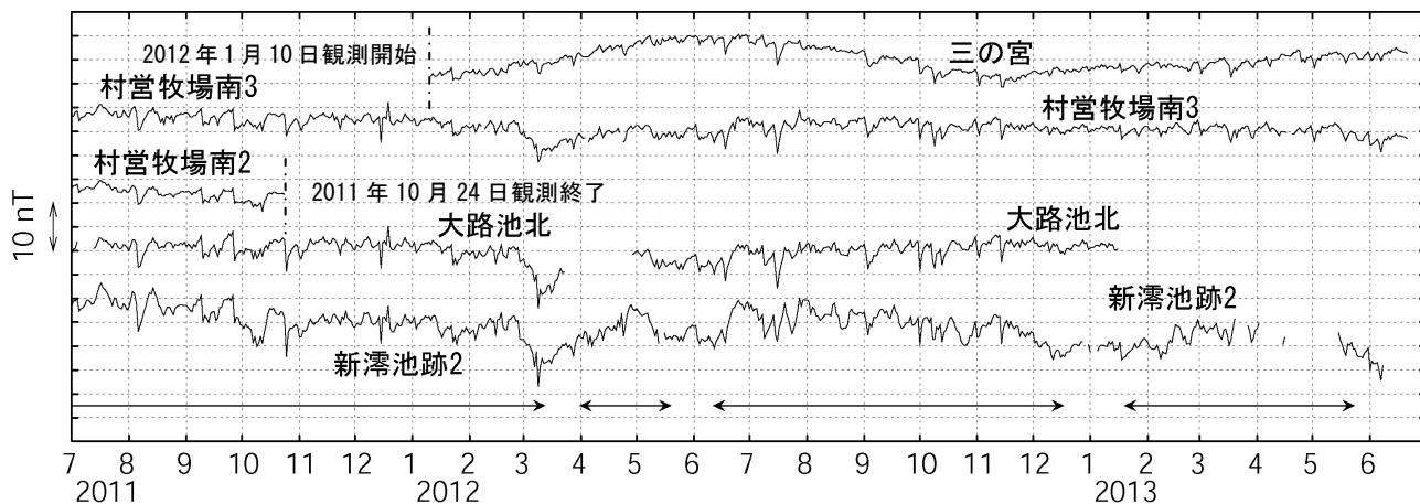
図 4 三宅島 全磁力連続観測による全磁力値の変化（2011 年 7 月～2013 年 6 月） 基準点：雄山北東
