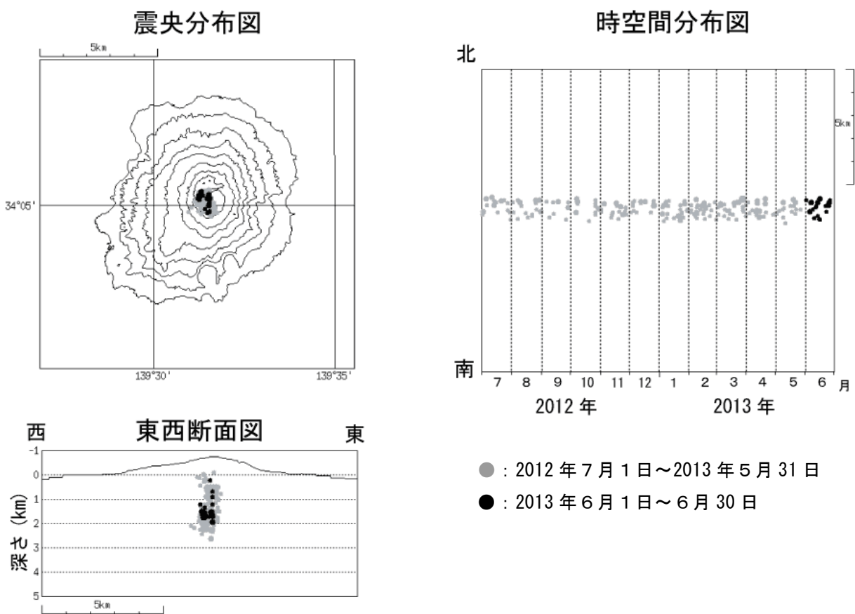
図5 三宅島 震源分布図（2012 年 7 月 1 日～2013 年 6 月 30 日）
