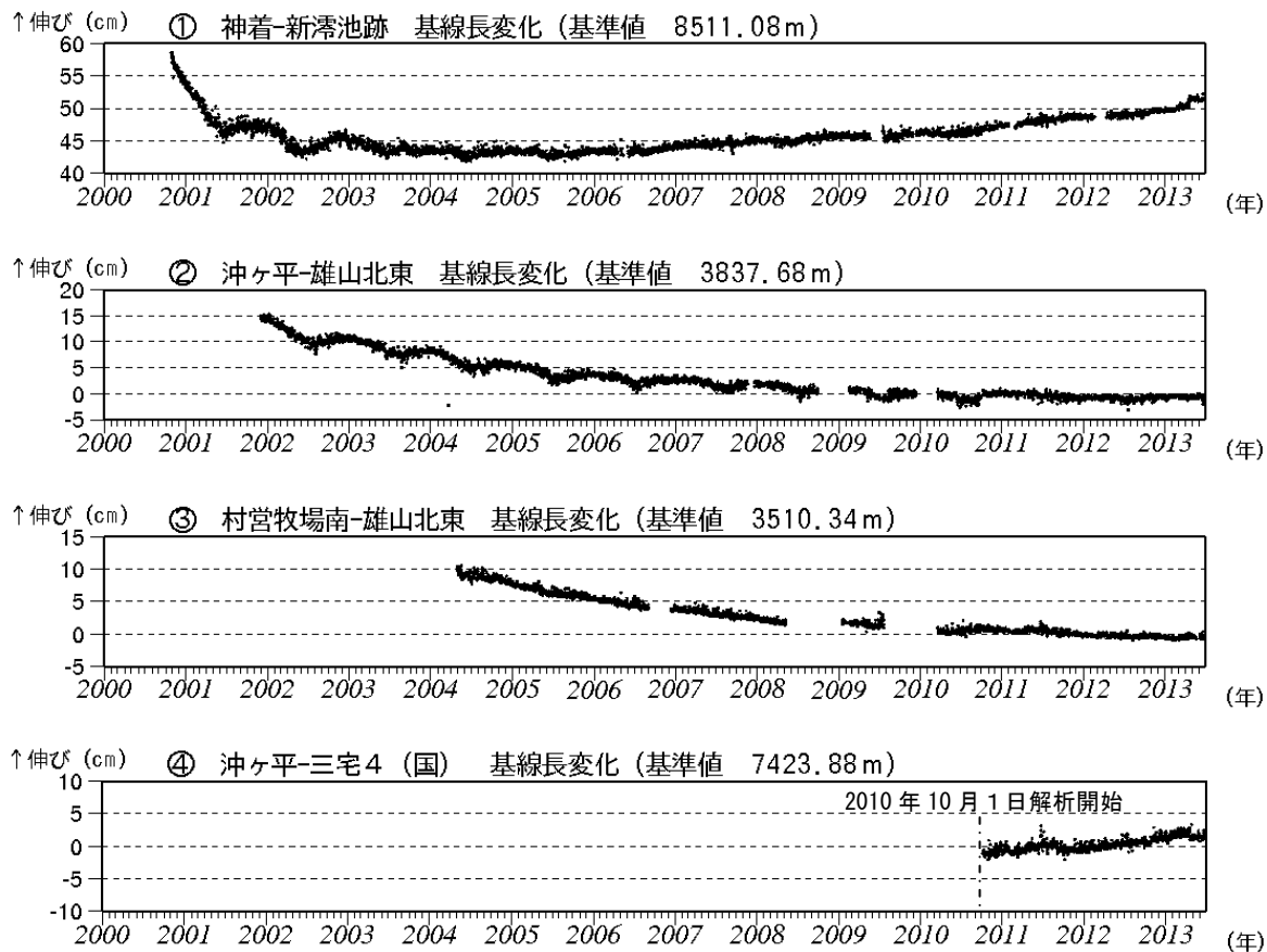
図 3 三宅島 GPS 連続観測結果（2000 年 1 月～2013 年 6 月）（国）：国土地理院 ・基線①～④は図 7（観測点配置図）の①～④にそれぞれ対応します。 ・グラフの空白部分は欠測を示します。 ・2010 年 10 月以降のデータについては、電離層の影響を補正する等、解析方法を改良しています。
