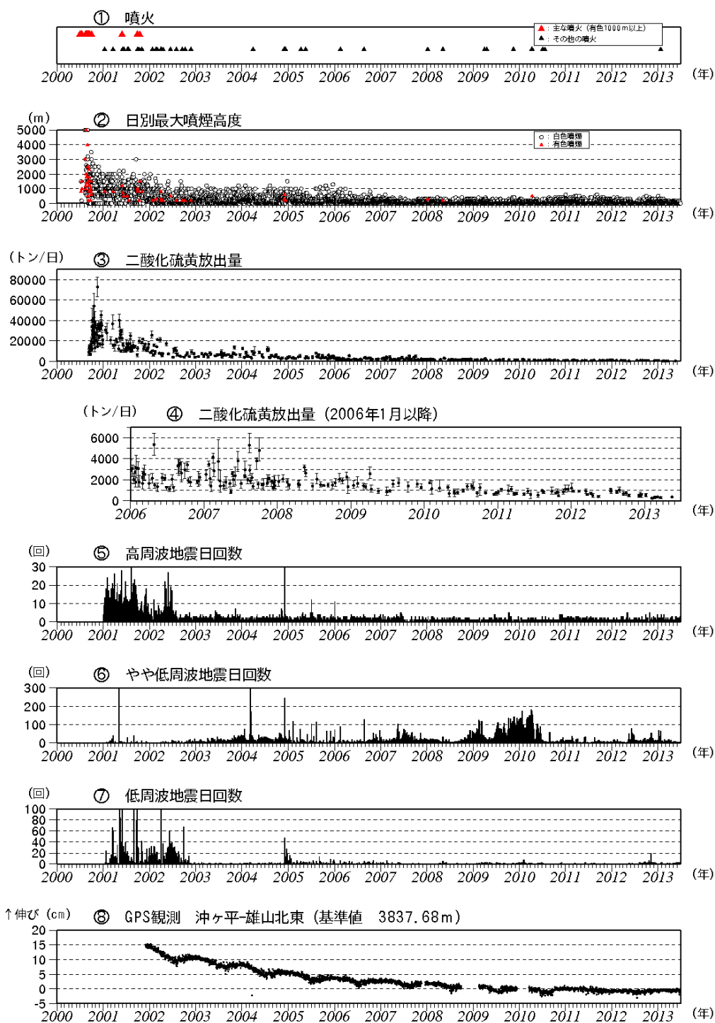
図 2 三宅島 最近の火山活動の経過図（2000 年 1 月～2013 年 6 月）
