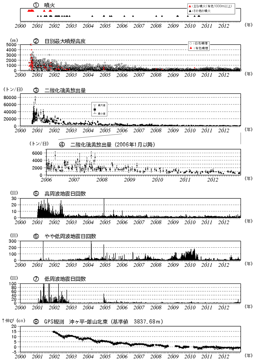
図2 三宅島 最近の火山活動の経過図 (2000年1月~2012年12月)
