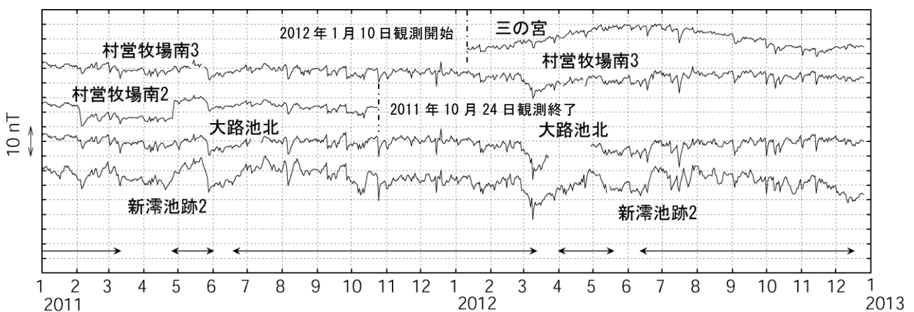
図 4 三宅島 全磁力連続観測による全磁力値の変化 (2011 年 1 月～2012 年 12 月) 基準点 : 雄山北東
