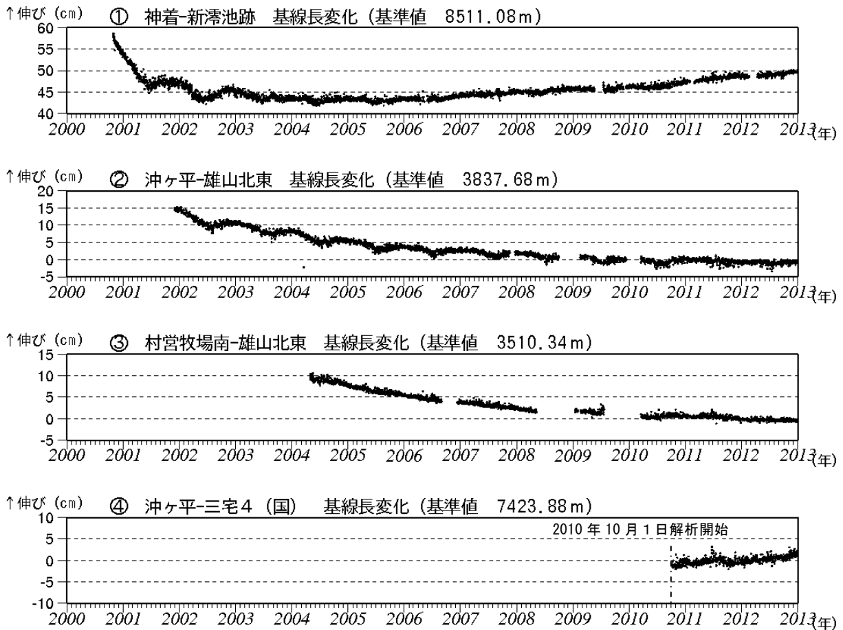
図 3* 三宅島 GPS 連続観測結果 (2000 年 1 月～2012 年 12 月) (国) : 国土地理院 基線①～④*は図 7 (観測点配置図) の①～④にそれぞれ対応します。 グラフの空白部分は欠測を示します。 2010 年 10 月以降のデータについては、電離層の影響を補正する等、解析方法を改良しています。
