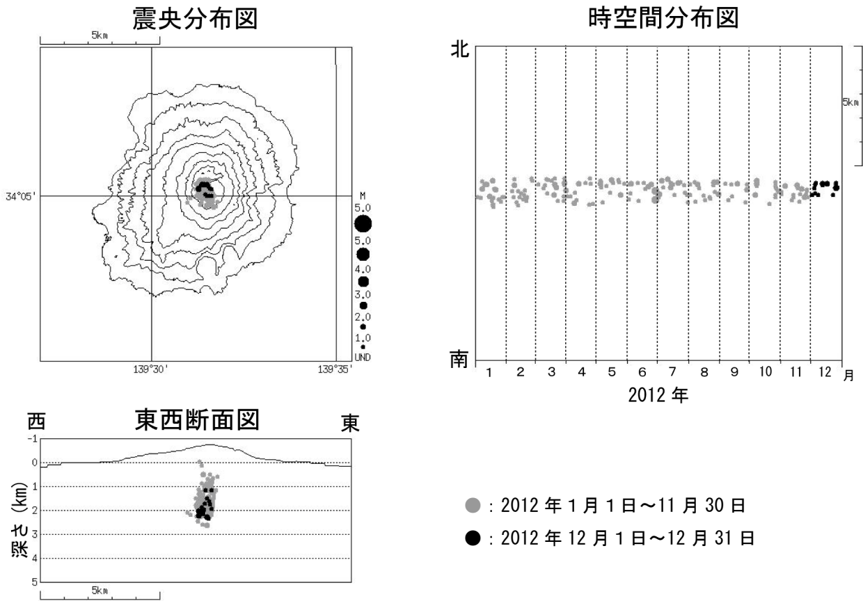
図 5※ 三宅島 震源分布図（2012 年 1 月 1 日～12 月 31 日）
