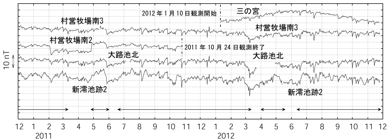
図4 三宅島 全磁力連続観測による全磁力値の変化（2010年12月～2012年11月）
