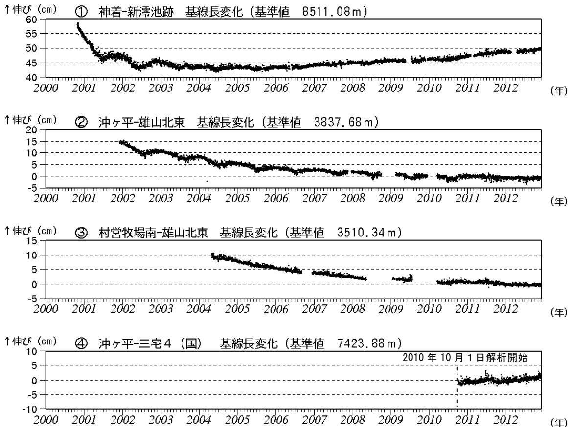
図3 三宅島 GPS 連続観測結果（2000年1月～2012年11月）（国）：国土地理院 基線①～④*は図7（観測点配置図）の①～④にそれぞれ対応します。 グラフの空白部分は欠測を示します。 2010年10月以降のデータについては、電離層の影響を補正する等、解析方法を改良しています。
