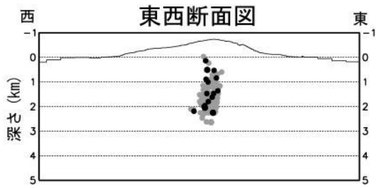
図 5※ 三宅島 震源分布図 (2011 年 12 月 1 日 ~ 2012 年 11 月 30 日)
