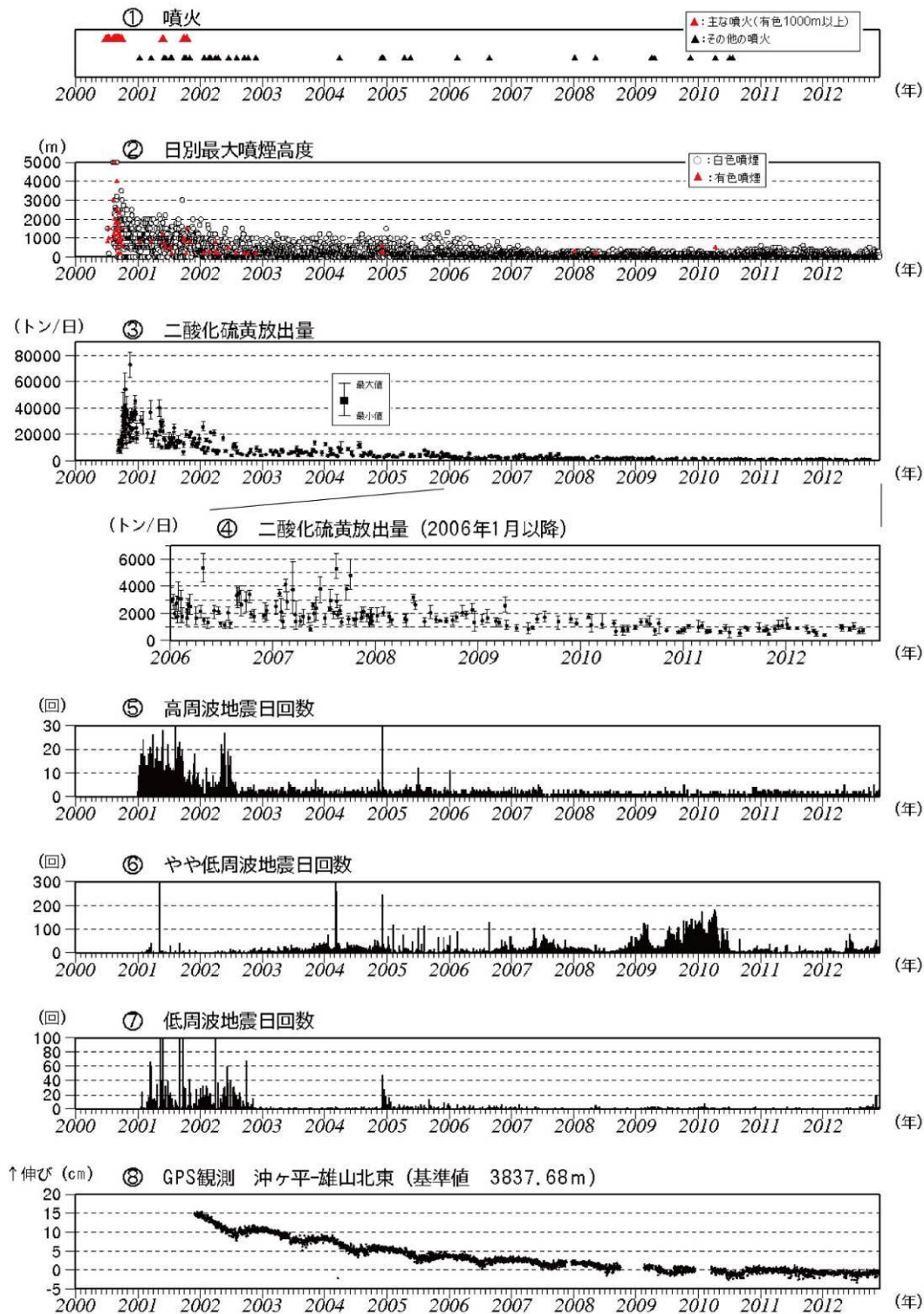
図 2 三宅島 最近の火山活動の経過図（2000 年 1 月～2012 年 11 月）
