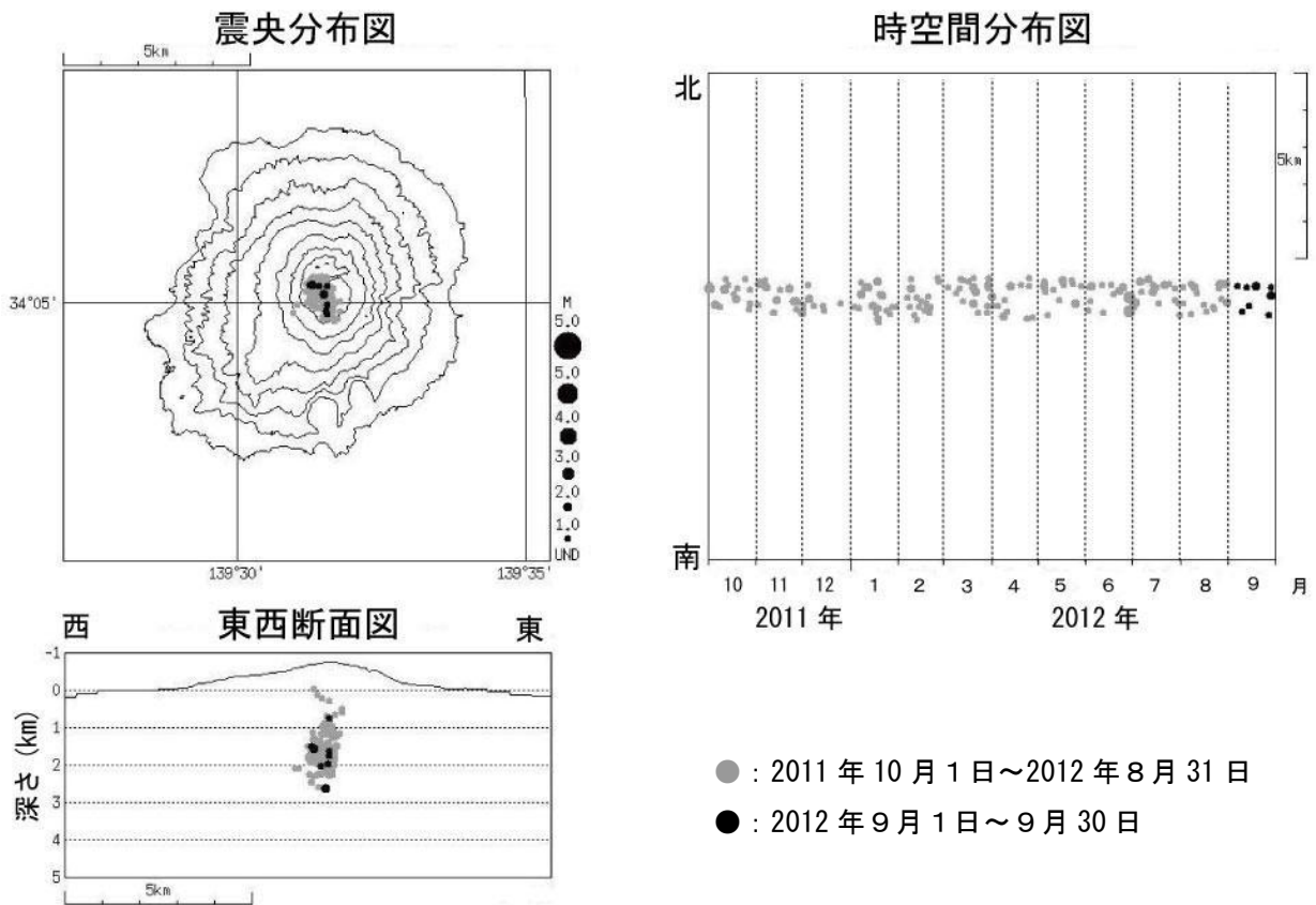
図 5* 三宅島 震源分布図（2011 年 10 月 1 日～2012 年 9 月 30 日）
