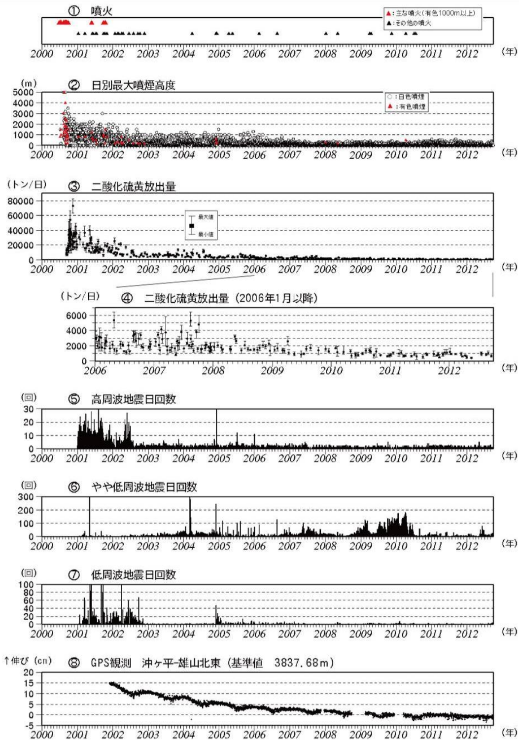
図 2 三宅島 最近の火山活動の経過図（2000 年 1 月～2012 年 9 月）
