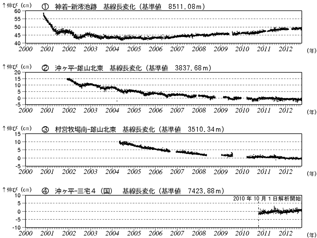
図3 三宅島 GPS 連続観測結果（2000 年 1 月～2012 年 9 月）（国）：国土地理院 基線①～④*は図7（観測点配置図）の①～④にそれぞれ対応します。 グラフの空白部分は欠測を示します。 2010 年 10 月以降のデータについては、電離層の影響を補正する等、解析方法を改良しています。
