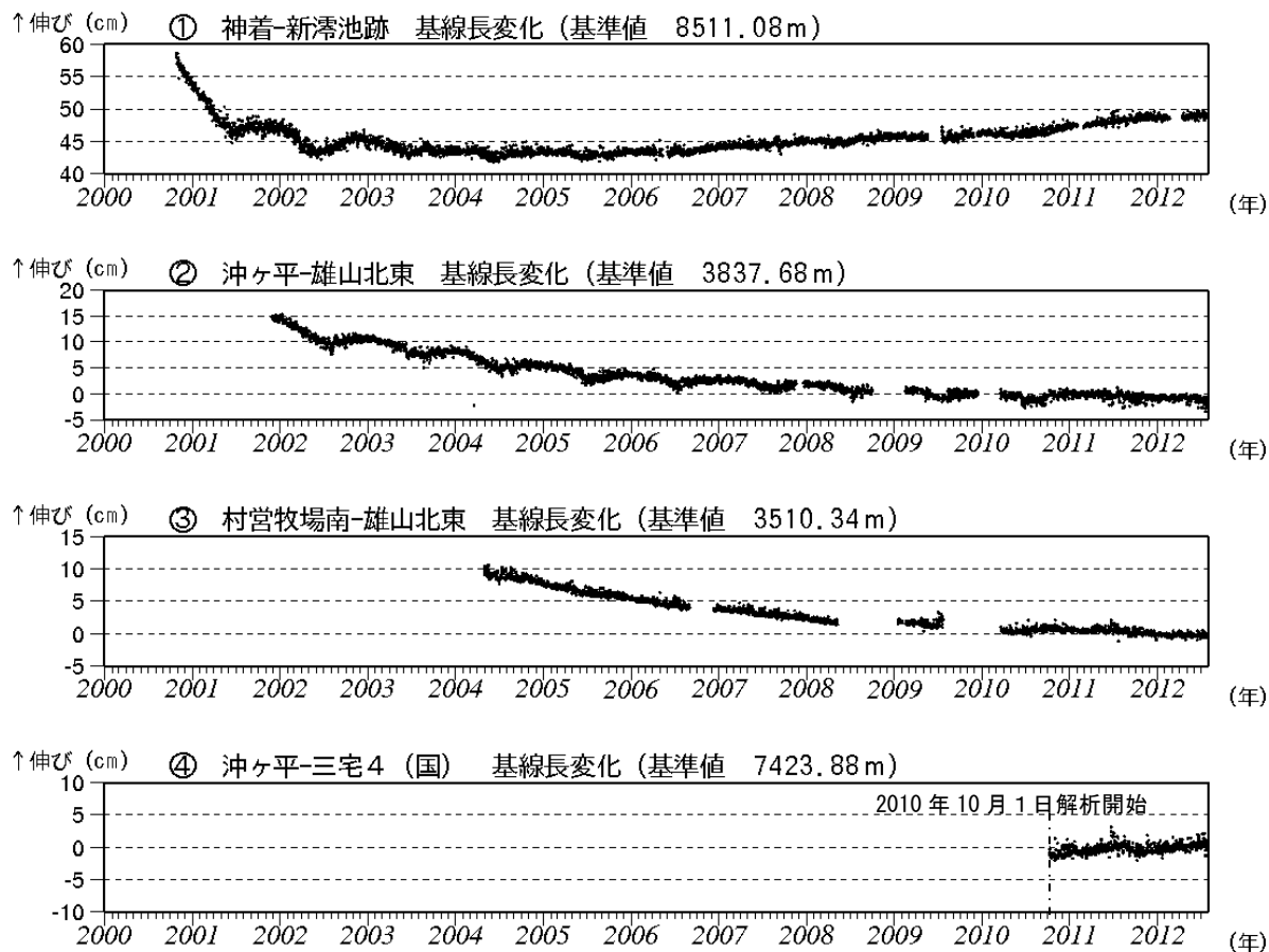
図3 三宅島 GPS 連続観測結果（2000 年 1 月～2012 年 7 月）（国）：国土地理院 基線①～④*は図7（観測点配置図）の①～④にそれぞれ対応します。 グラフの空白部分は欠測を示します。 2010 年 10 月以降のデータについては、電離層の影響を補正する等、解析方法を改良しています。
