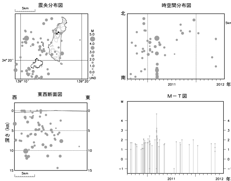
図4* 新島 広域地震観測網による山体・周辺の地震活動 (2010年8月1日~2012年7月31日)
