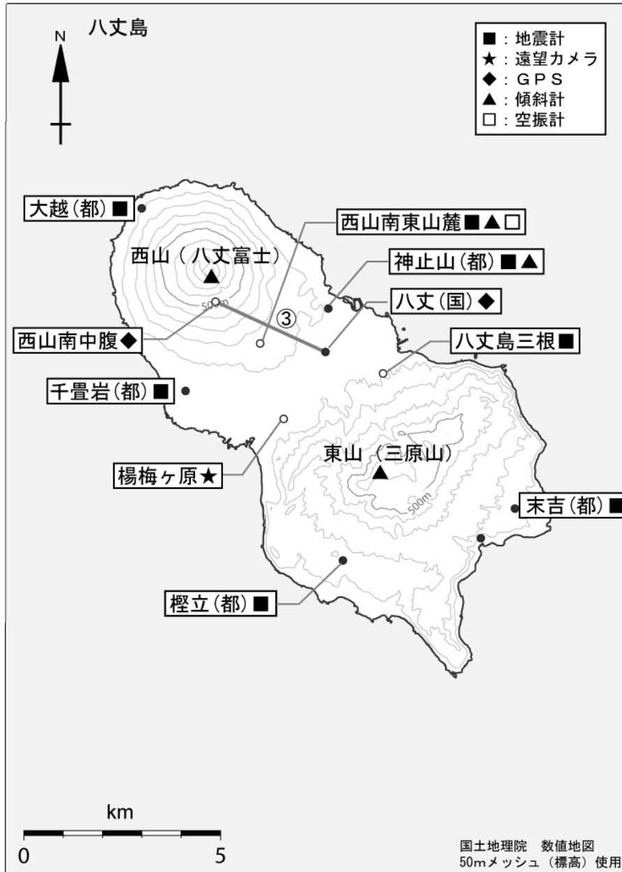
図3 八丈島 観測点配置図 GPS 基線③は図2の③*に対応しています。
