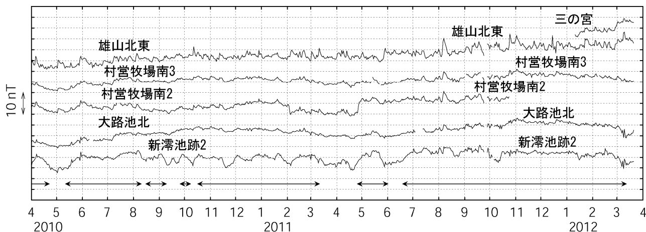
図6 三宅島 全磁力連続観測による全磁力値の変化 (2010年4月~2012年3月)
