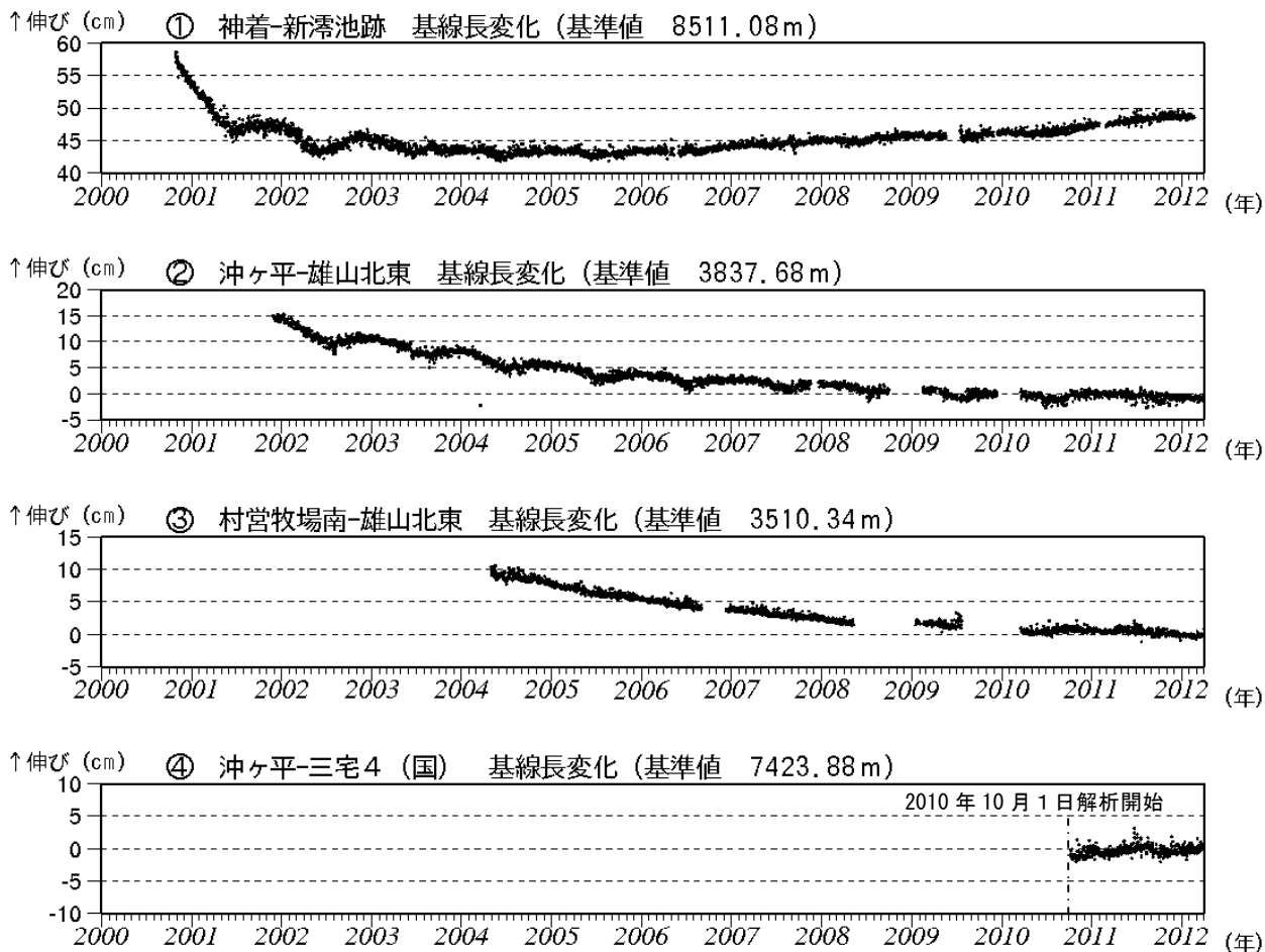
図5 三宅島 GPS 連続観測結果 (2000年~2012年3月) (国): 国土地理院
