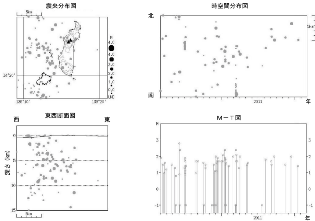
図4* 新島 広域地震観測網による山体・周辺の地震活動(2010年3月1日~2012年2月29日)
