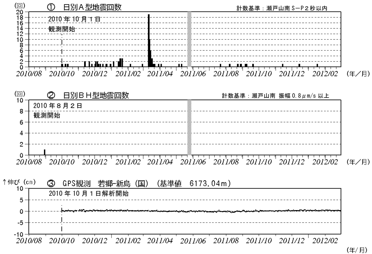
図3 新島 火山活動経過図(2010年8月~2012年2月)
