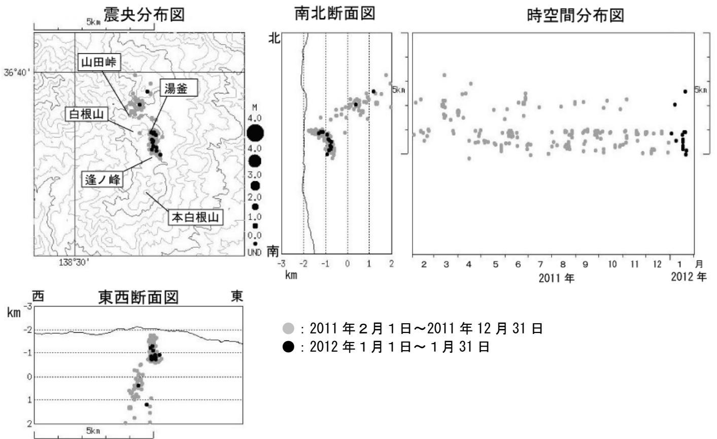
図4※ 草津白根山 震源分布図 (2011年2月1日~2012年1月31日)
