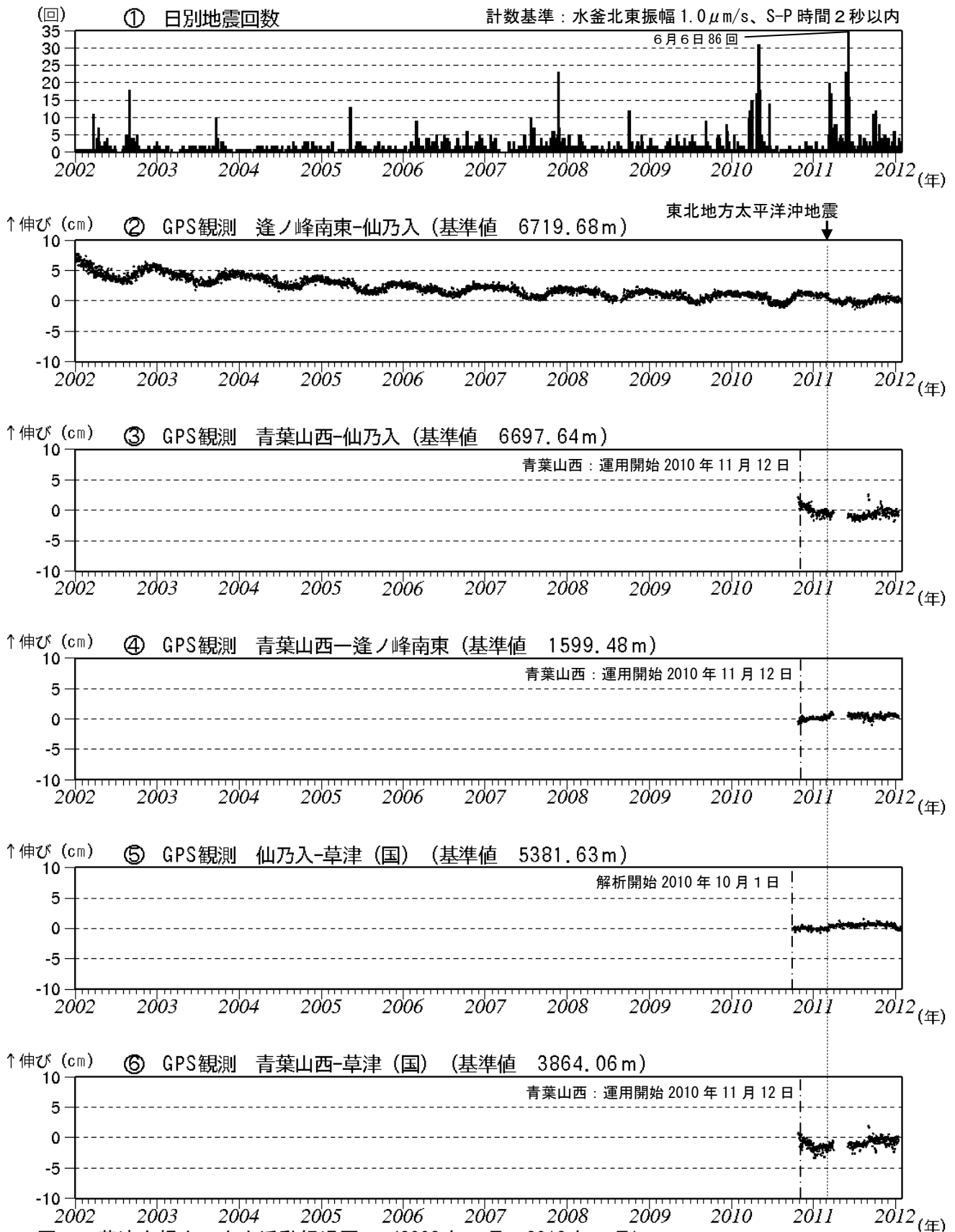
図5 草津白根山 火山活動経過図 (2002年1月~2012年1月)
