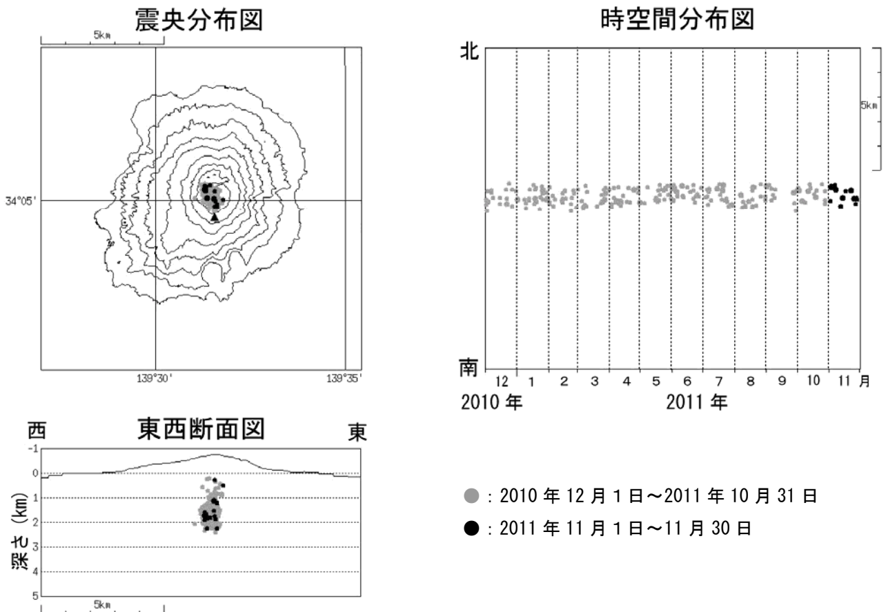
図4※ 三宅島 震源分布図 (2010 年 12 月 1 日～2011 年 11 月 30 日)
