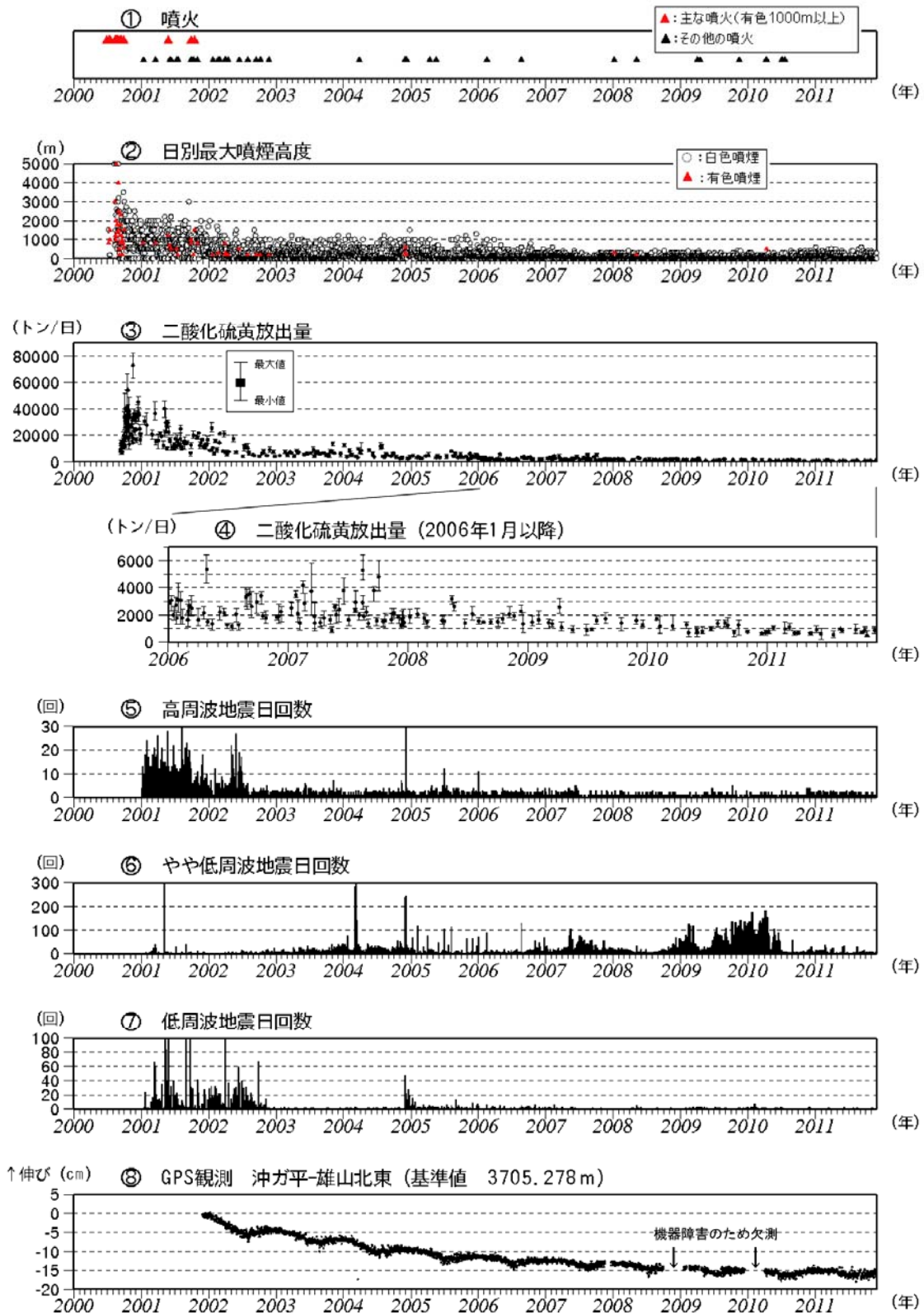
図2 三宅島 最近の火山活動の推移 (2000年1月~2011年11月)
