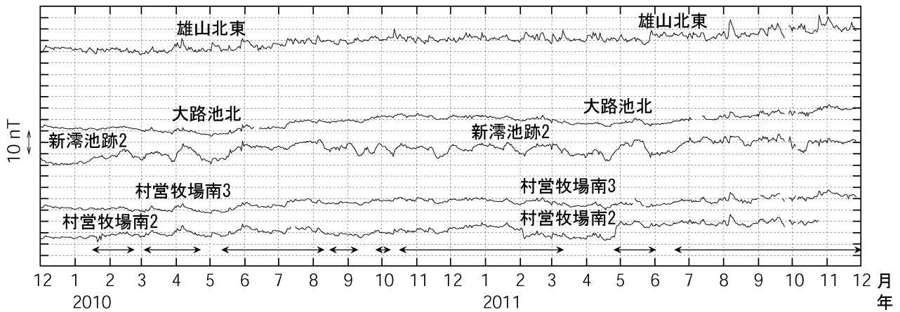
図3 三宅島 全磁力連続観測による全磁力値の変化 (2009 年 12 月～2011 年 11 月) ←→で示した期間の全磁力値は三宅島周辺の海流の影響を受けていると推測されます。 nT (ナノテスラ) は磁場の強さを表す単位です。
