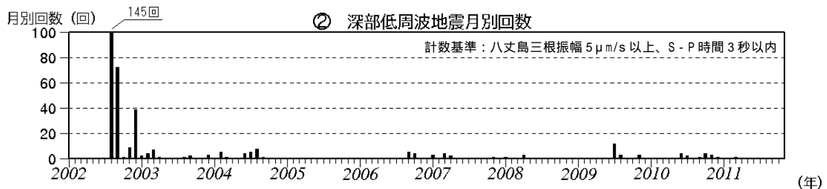
図 2 八丈島 月別地震回数（2002 年 1 月～2011 年 10 月）
