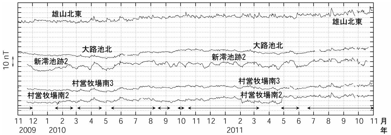
図3 三宅島 全磁力連続観測による全磁力値の変化(2009年11月~2011年10月) ←→で示した期間の全磁力値は三宅島周辺の海流の影響を受けていると推測されます。 nT(ナノテスラ)は磁場の強さを表す単位です。
