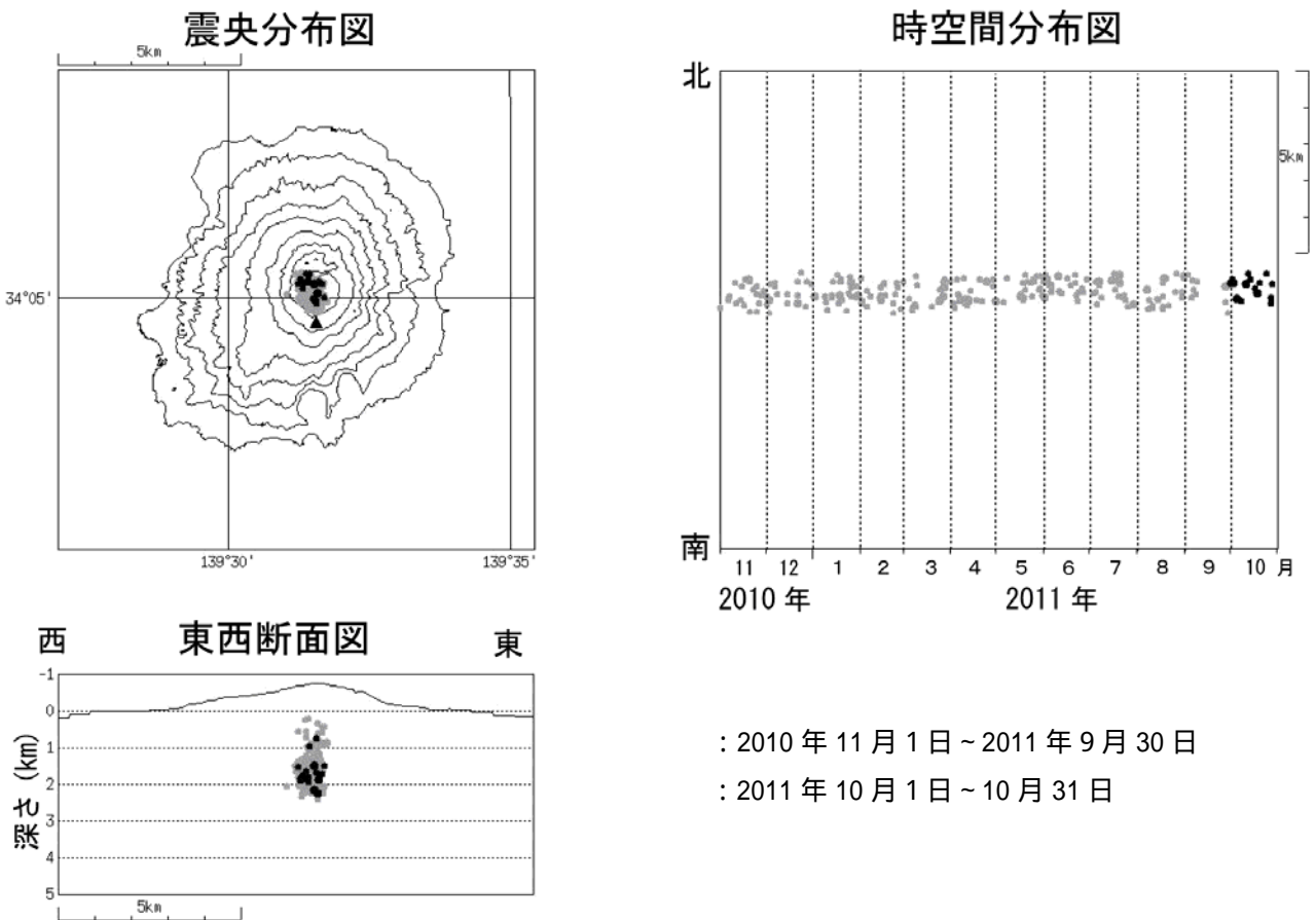
図4 三宅島 震源分布図(2010年11月1日~2011年10月31日)
