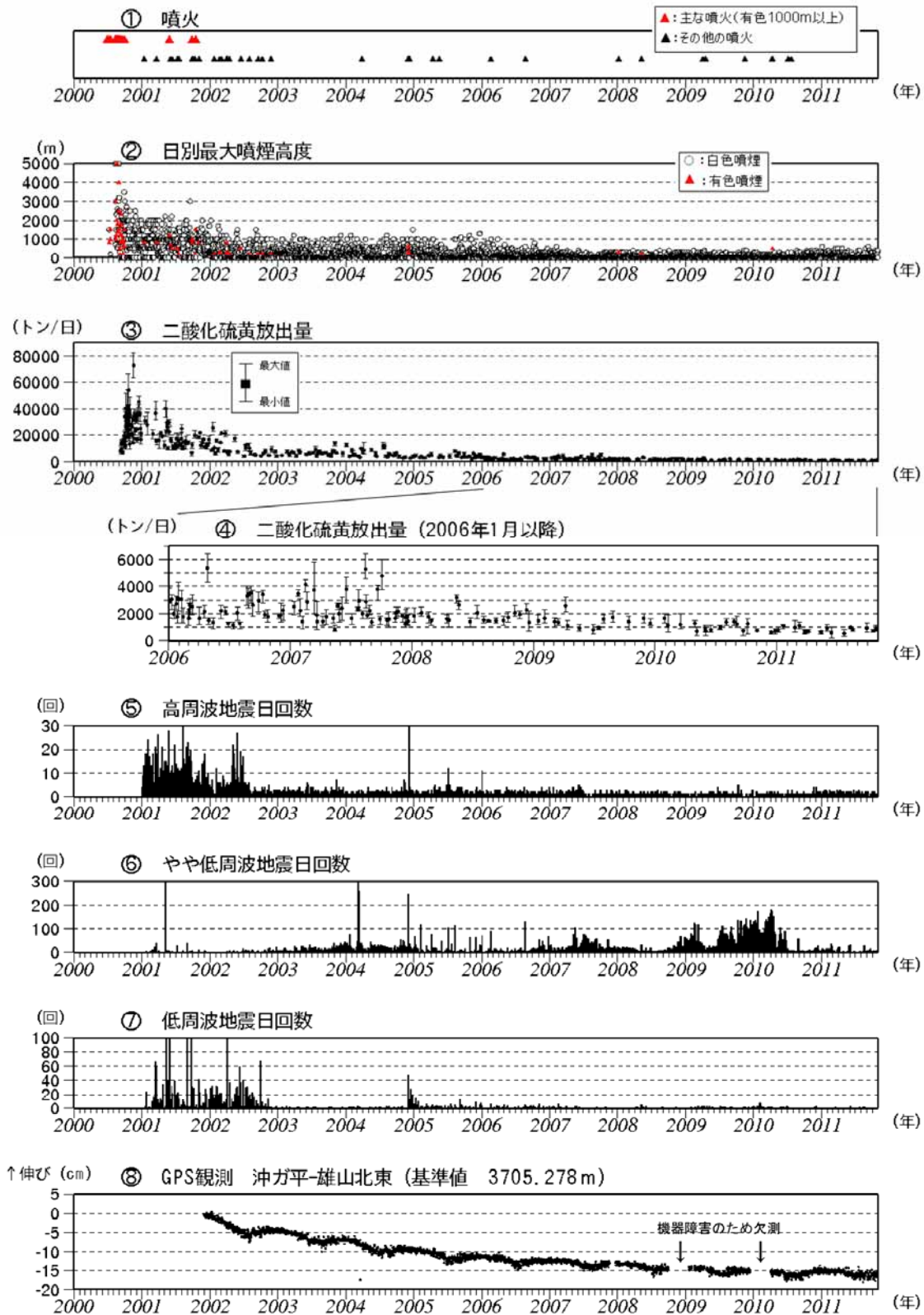
図2 三宅島 最近の火山活動の推移(2000年1月~2011年10月)
