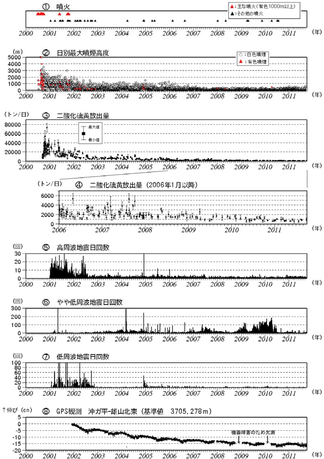
図2 三宅島 最近の火山活動の推移 (2000年1月～2011年9月)
