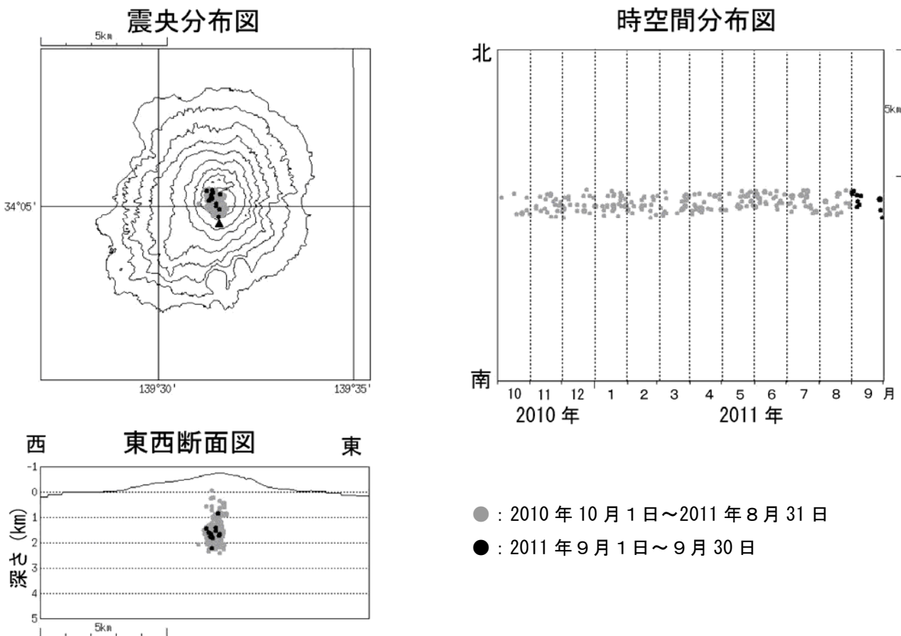
図4※ 三宅島 震源分布図 (2010年10月1日～2011年9月30日)
