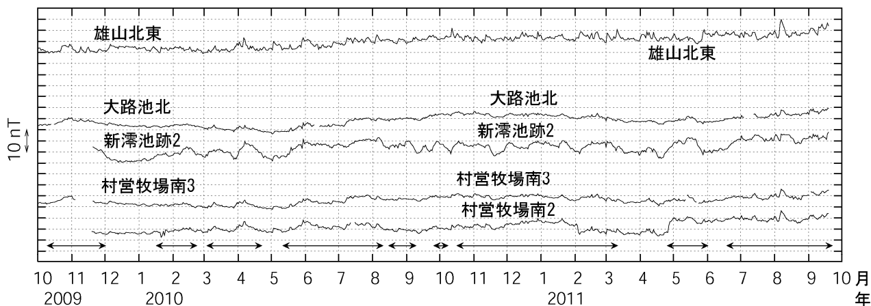
図3 三宅島 全磁力連続観測による全磁力値の変化 (2009年10月～2011年9月) ←→で示した期間の全磁力値は三宅島周辺の海流の影響を受けていると推測されます。 2011年8月上旬に全観測点で見られる変動は磁気嵐の影響と考えられます。 nT (ナノテスラ) は磁場の強さを表す単位です。
