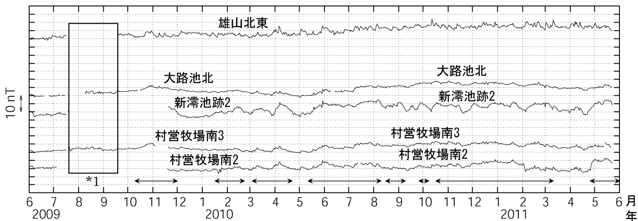
図3 三宅島 全磁力連続観測による全磁力値の変化 (2009年6月~2011年5月24日) ←→で示した期間の全磁力値は三宅島周辺の海流の影響を受けていると推測されます。 nT (ナノテスラ) は磁場の強さを表す単位です。
