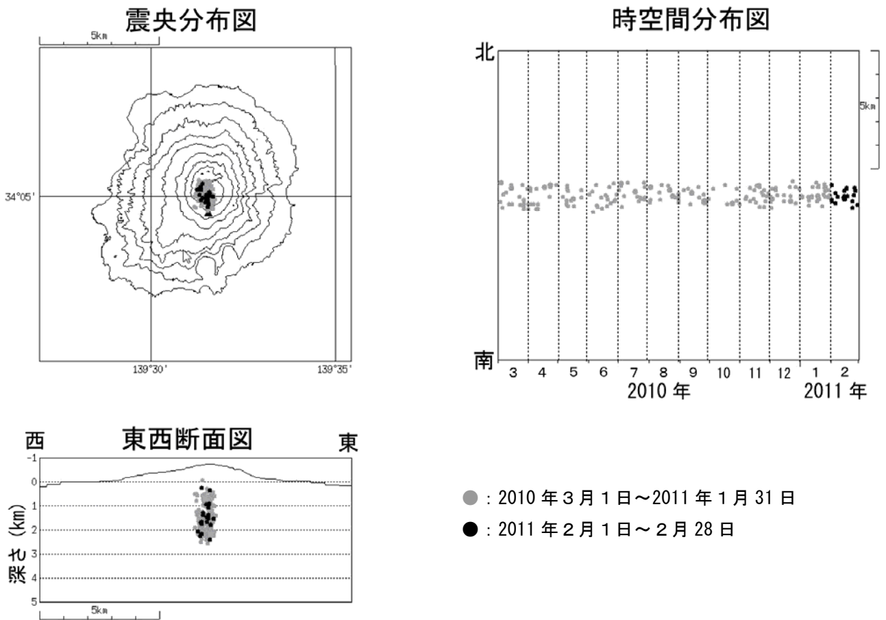
図4※ 三宅島 震源分布図 (2010年3月1日~2011年2月28日)
