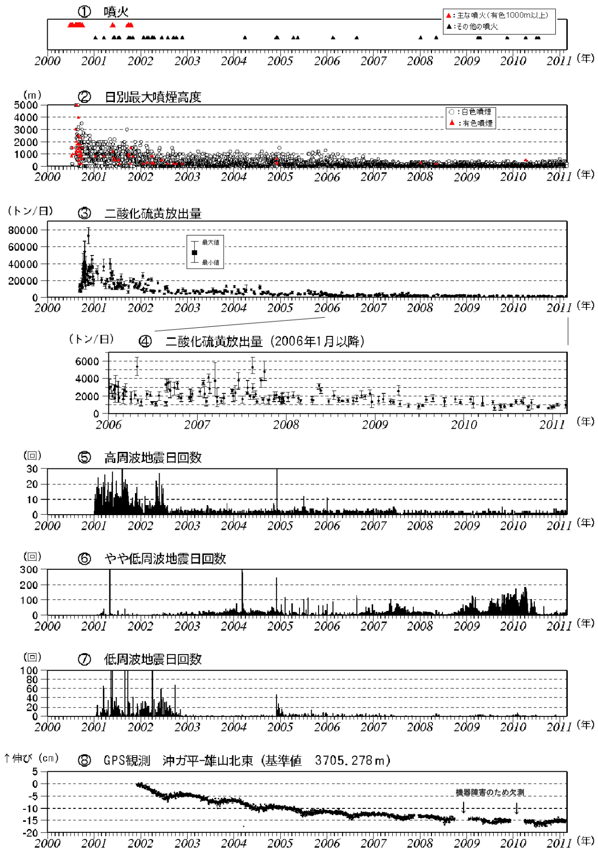
図2 三宅島 最近の火山活動の推移 (2000年1月~2011年2月)
