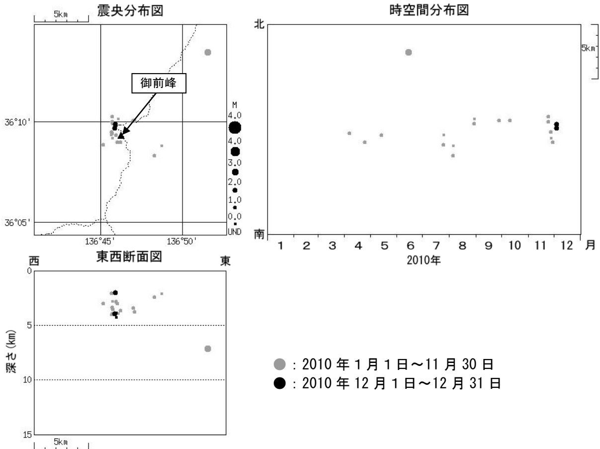
図 3※ 白山 震源分布図（2010 年 1 月 1 日～12 月 31 日） M（マグニチュード）は地震の規模を表します。 図中の震源要素は一部暫定値で、後日変更することがあります。
