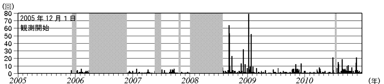
図 2 白山 日別地震回数（2005 年 12 月 1 日～2010 年 12 月 31 日） 図の灰色部分は機器障害のため欠測
