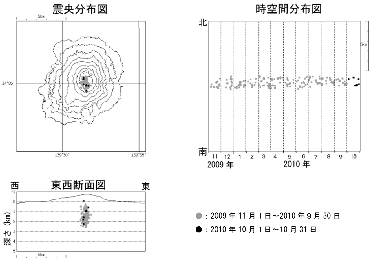
図4※ 三宅島 震源分布図 (2009年11月1日~2010年10月31日)
