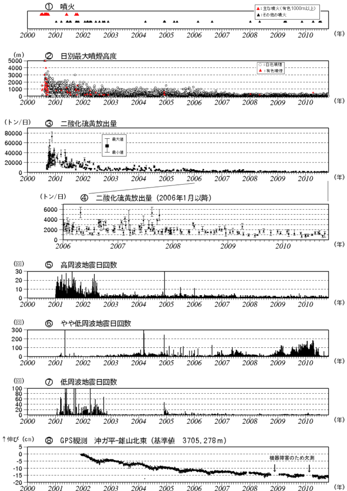
図2 三宅島 最近の火山活動の推移 (2000年1月～2010年10月)
