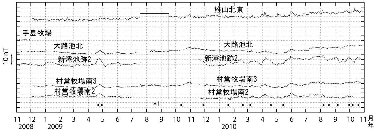
図3 三宅島 全磁力連続観測による全磁力値の変化 (2008年10月~2010年10月31日) ←→で示した期間の全磁力値は三宅島周辺の海流の影響を受けていると推測されます。 nT (ナノテスラ) は磁場の強さを表す単位です。
