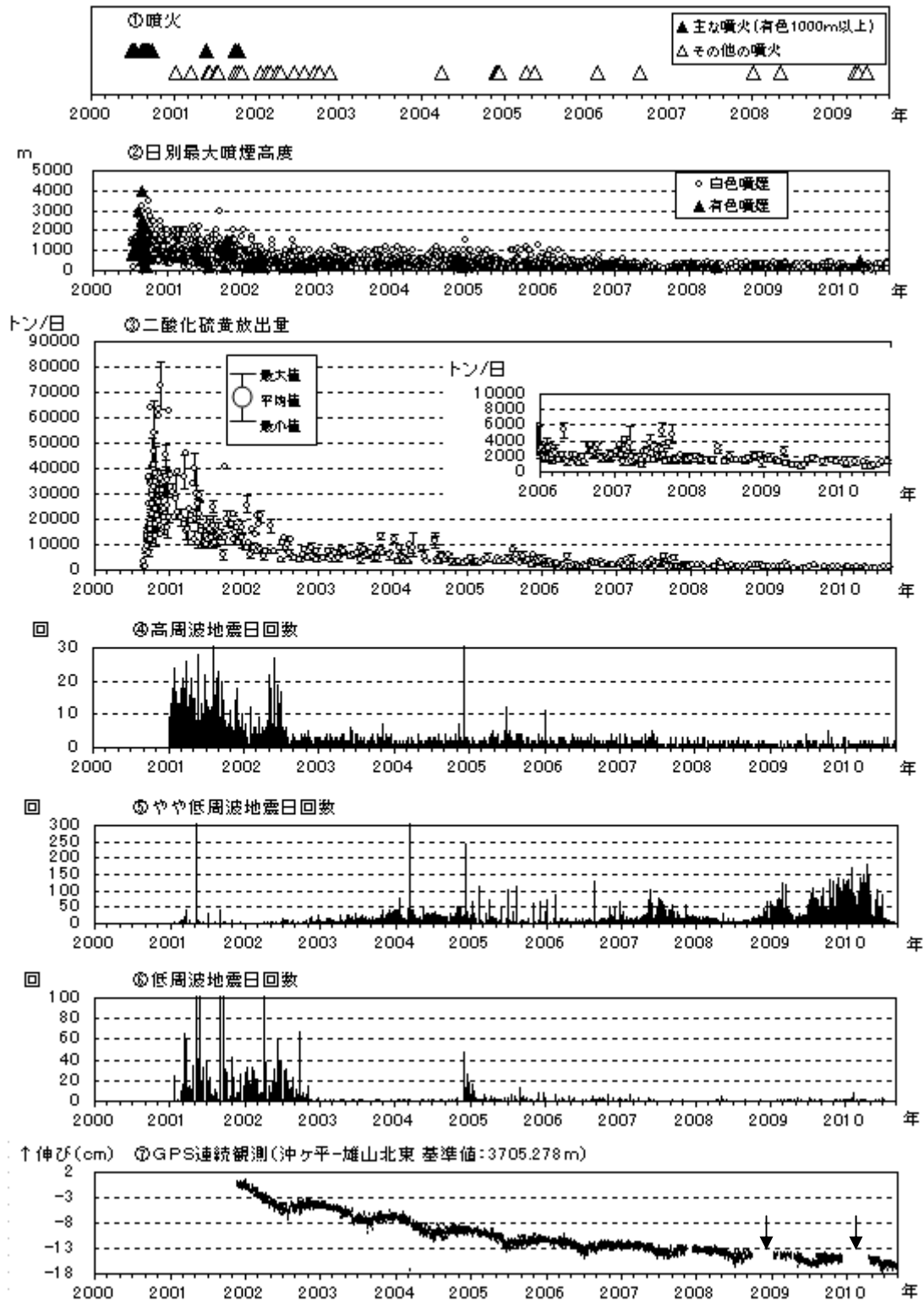
図2 三宅島 最近の火山活動の推移（2000年1月～2010年8月）
