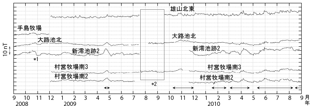
図3 三宅島 全磁力連続観測による全磁力値の変化 (2008年9月~2010年8月31日) ←→で示した期間の全磁力値は三宅島周辺の海流の影響を受けていると推測されます。 nT (ナノテスラ) は磁場の強さを表す単位です。
