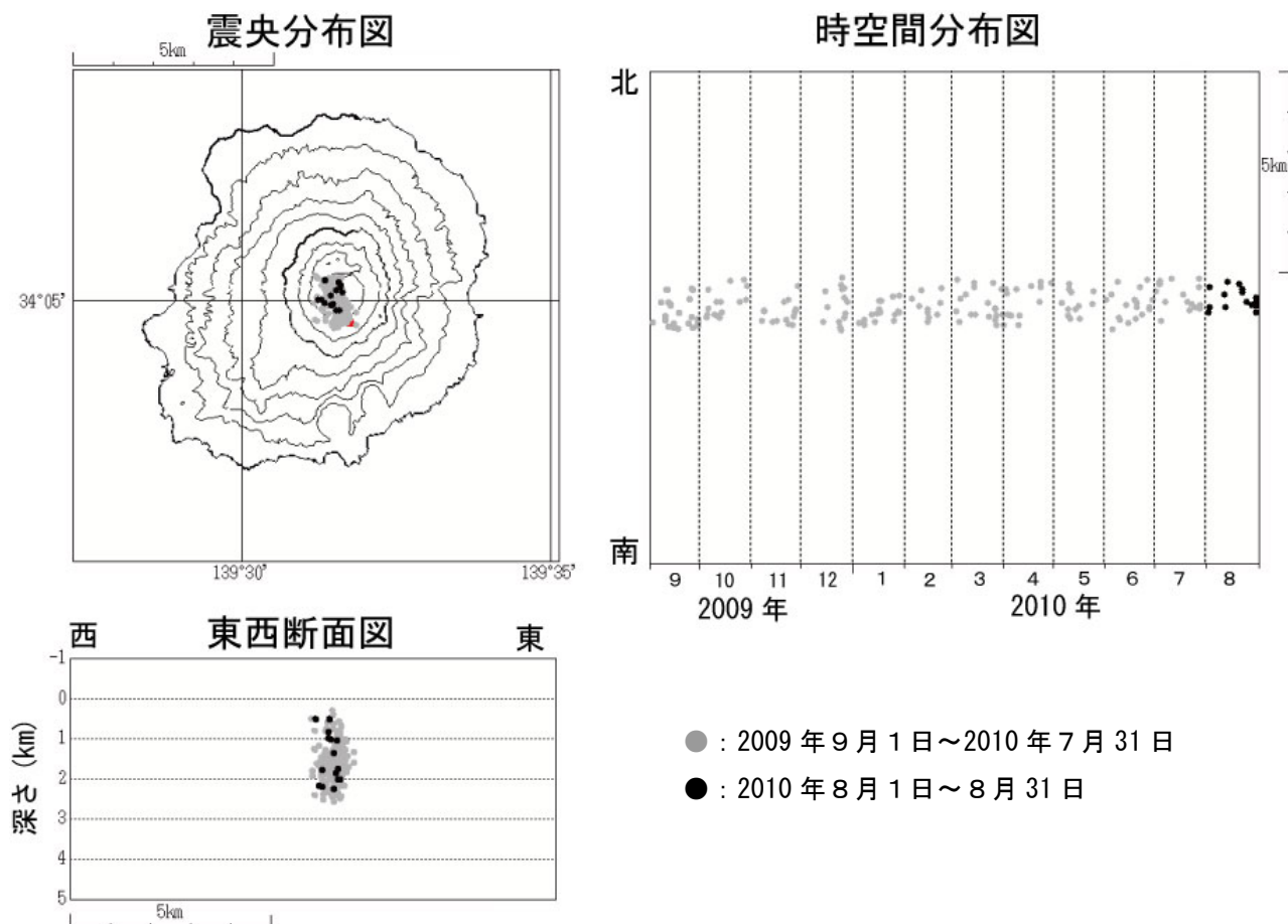
図4※ 三宅島 震源分布図 (2009年9月1日~2010年8月31日)
