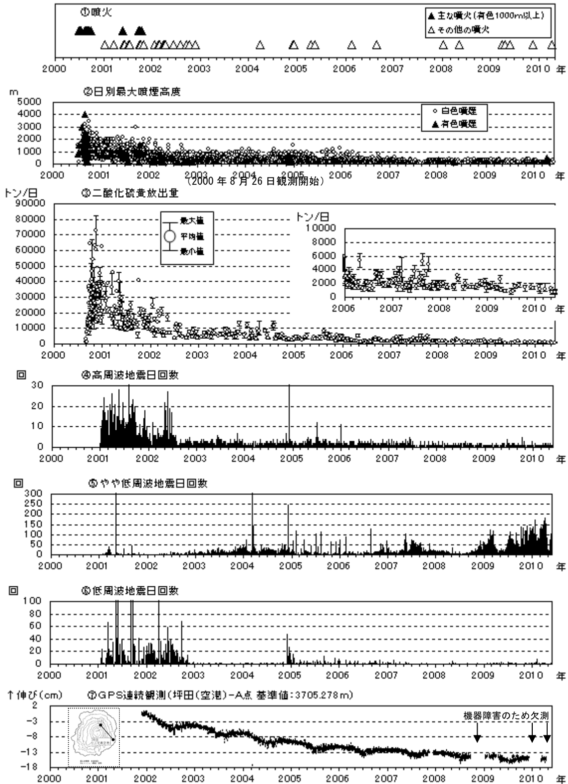
図2 三宅島 最近の火山活動の推移 (2000年1月～2010年5月)
