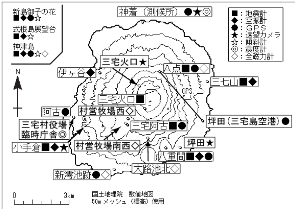
図 6 三宅島 気象庁の観測点配置図（小さな白丸は観測点位置を示しています） GPS 基線（A 点－坪田）は図 2 の⑦に対応しています。
