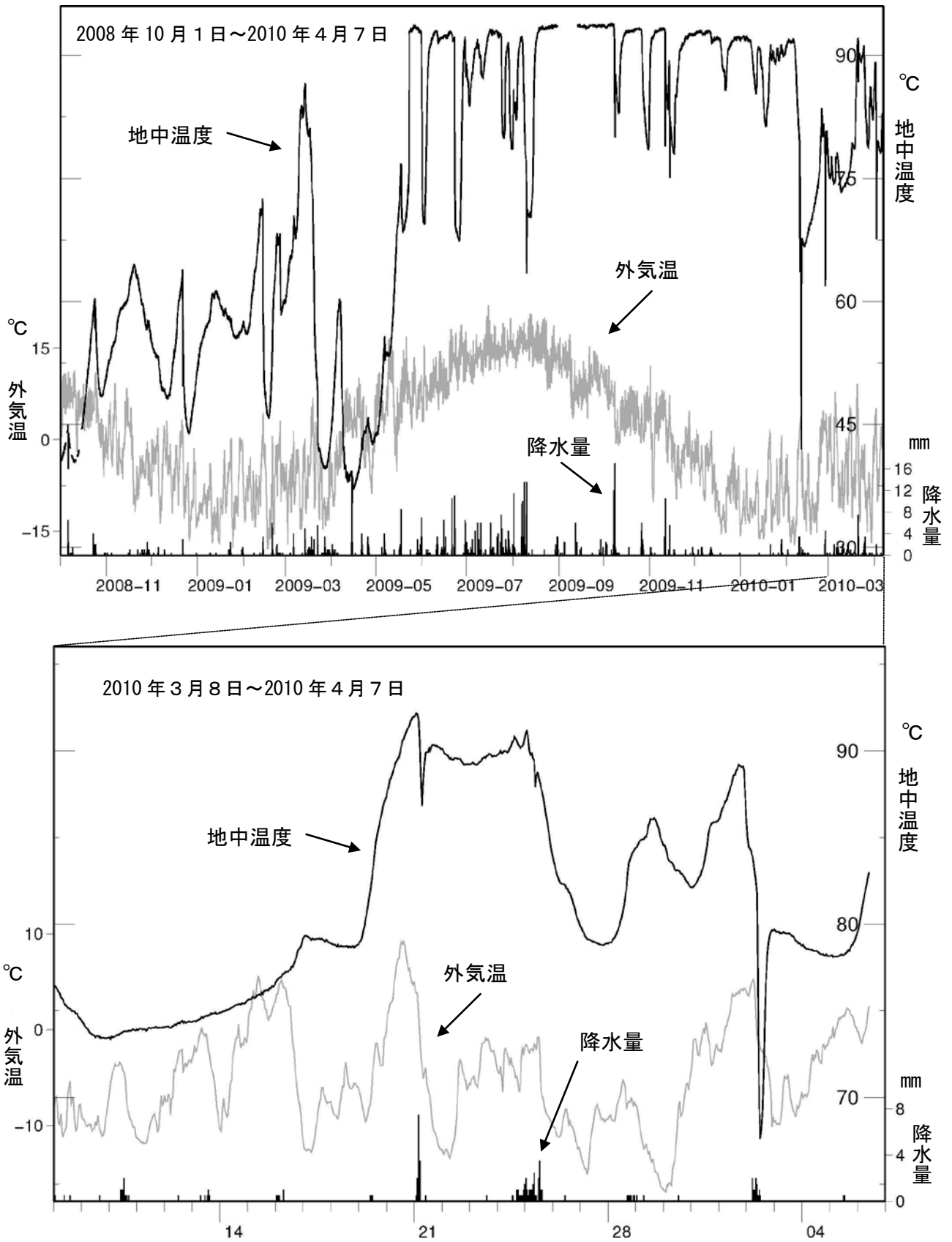
図 4※ 草津白根山 湯釜火口内北東部の噴気地帯 地中温度、外気温と降水量(湯釜内) (2008年10月1日～2010年4月7日、東京工業大学による) 上図：長期グラフ(2008年10月1日～2010年4月7日) 下図：短期グラフ(2010年3月8日～4月7日)
