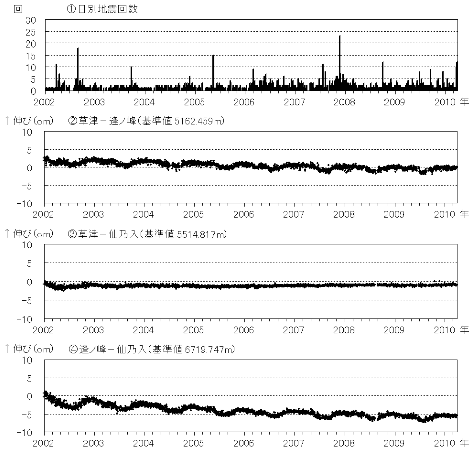
図 7 草津白根山 最近の火山活動の推移 (2002 年 1 月～2010 年 3 月)
