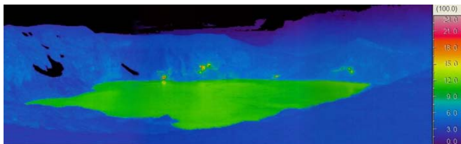
図 3 草津白根山 湯釜火口北壁の地表面温度分布 1) （湯釜火口南側から撮影、撮影場所は図 5 を参照） 今回（2010 年 3 月 19 日）の観測では日射の影響もみられます
