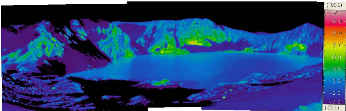
図 2 草津白根山 湯釜火口北壁の地表面温度分布 1) （北西側から撮影、撮影場所は図 5 を参照） 前回（2009 年 9 月 9 日）の観測では日射の影響もみられます
