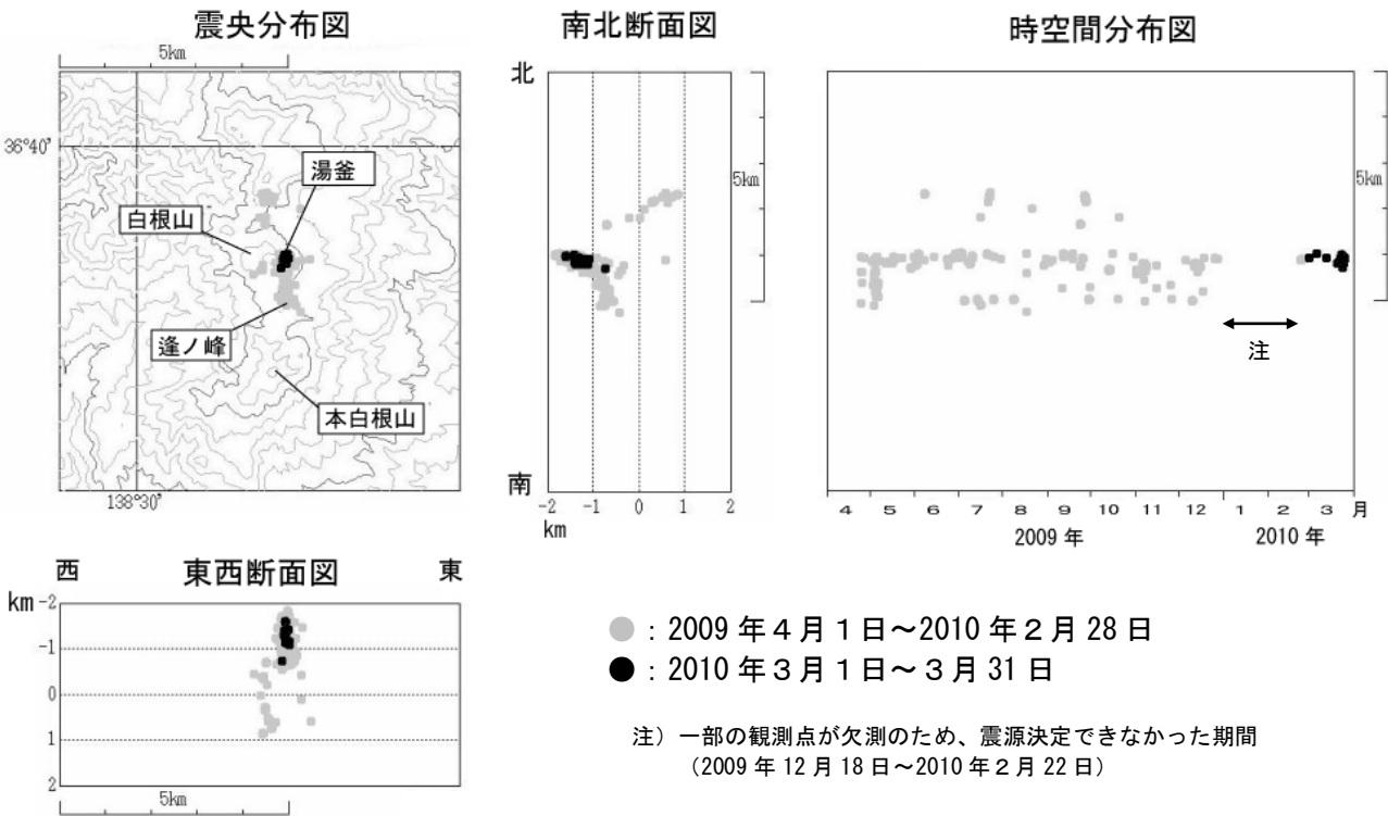
図 6※ 草津白根山 震源分布図 (2009 年 4 月 1 日～2010 年 3 月 31 日)
