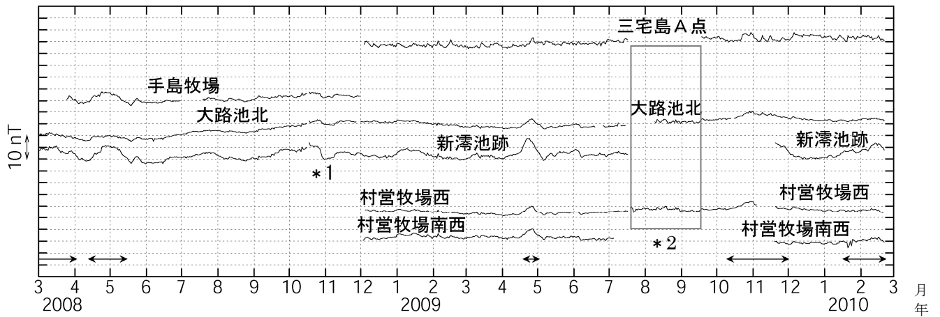
図 3 三宅島 全磁力連続観測による全磁力値の変化 (2008 年 3 月～2010 年 2 月 21 日)
