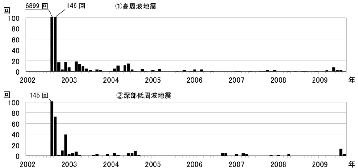
図1 八丈島 月別地震回数(2002年1月~2009年8月)
