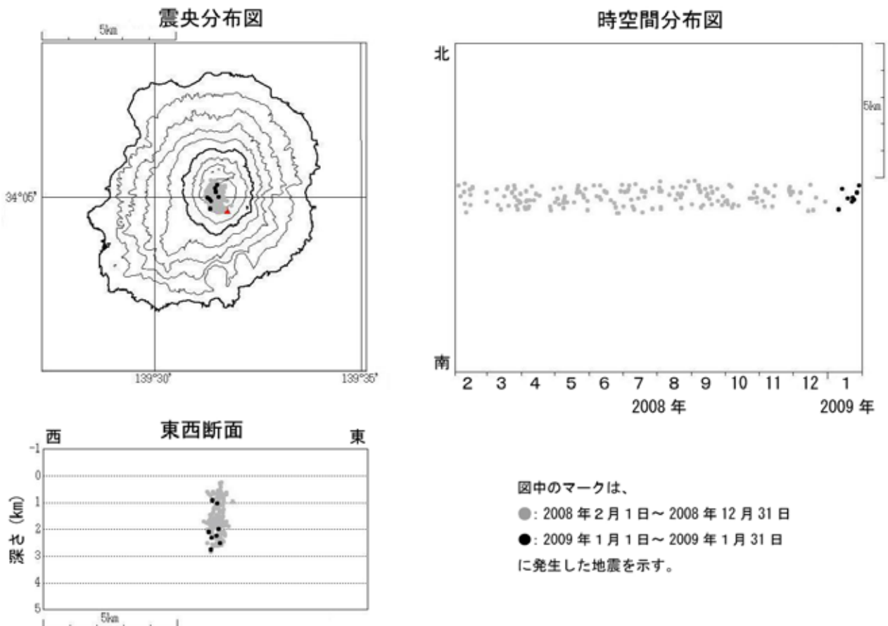
図4 三宅島 震源分布図(2008年2月1日~2009年1月31日)
