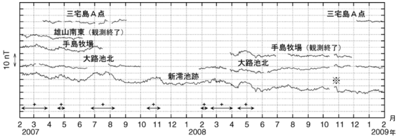
図3 三宅島 全磁力連続観測による全磁力値の変化(2007年1月~2009年1月) ←→で示した期間の全磁力値は三宅島周辺の海流の影響を受けていると推測されます。 nT(ナノテスラ)は磁場の強さを表す単位です。 2008年10月下旬の全磁力減少の原因は不明ですが、黒潮の流軸が離れていく場合に同様の傾向がみられます。
