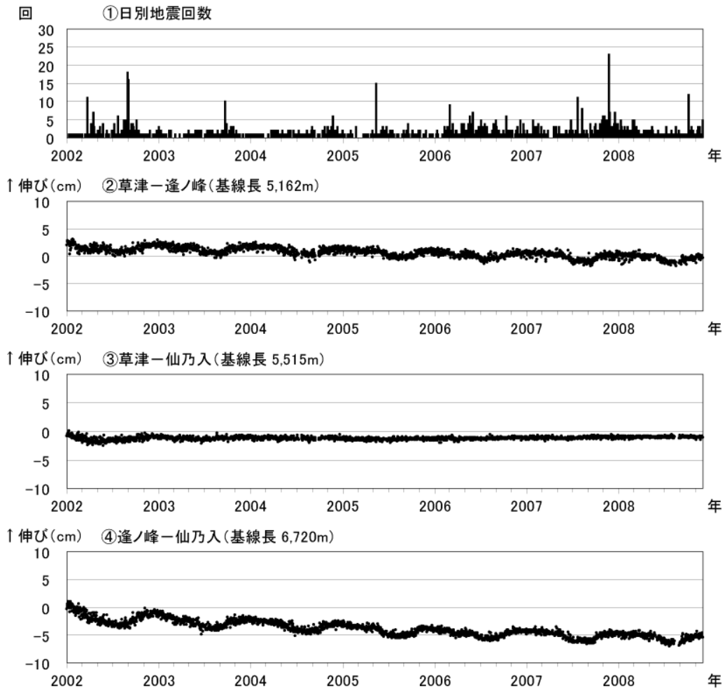
図8 草津白根山 最近の火山活動の推移(2002年1月~2008年11月) 山体付近に発生した地震の日別回数 ~ GPS連続観測による基線長変化 基線長変化にみられる冬季の伸びと夏季の縮みの傾向は季節変動による変化です。 ~ は図1の ~ に対応しています。
