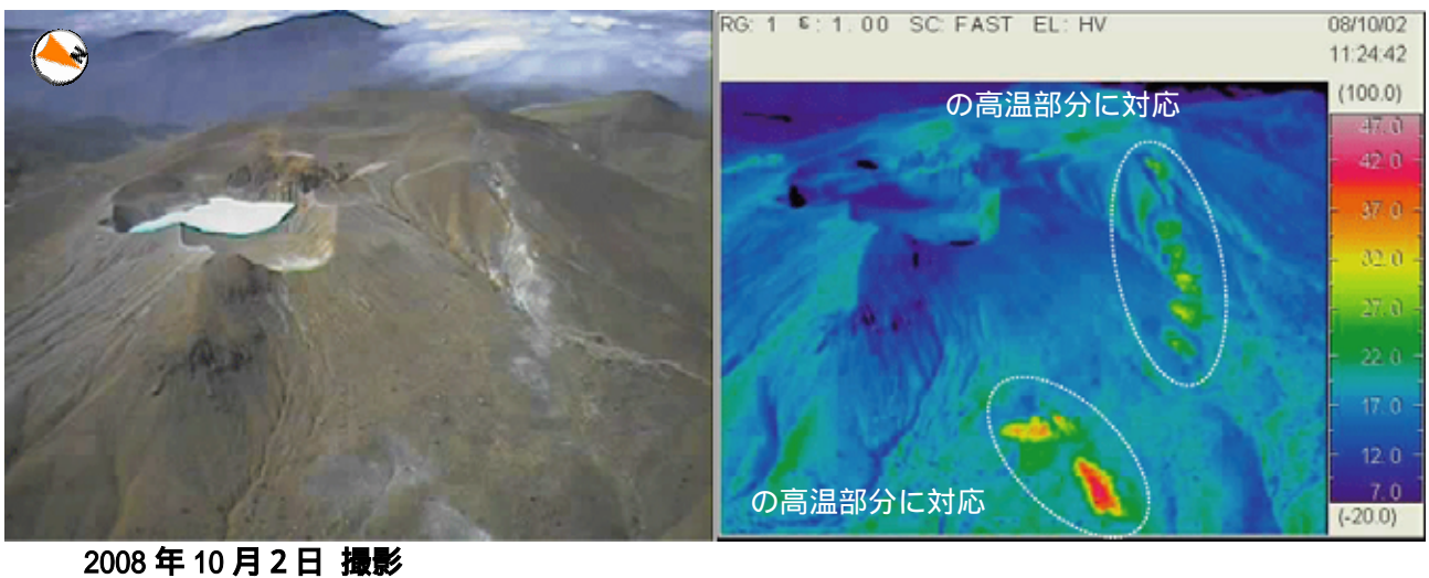
図5 草津白根山 北側噴気地帯と水釜火口北東斜面の噴気の状態及び地表面温度分布 ・ 高温領域の広がりには特段の変化はありませんでした。
