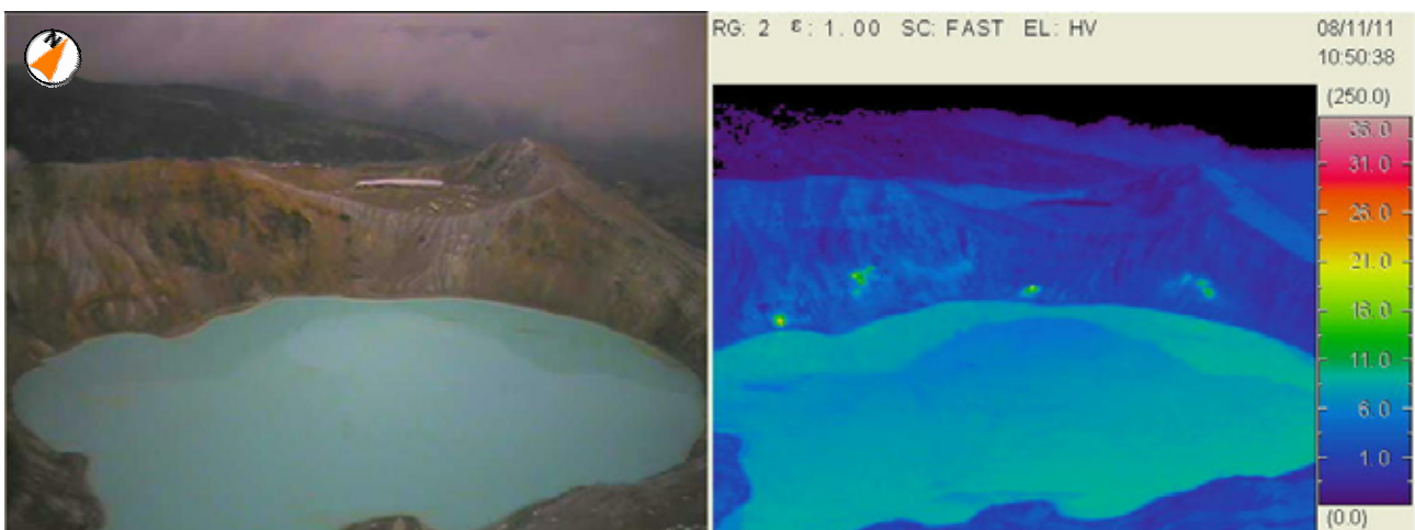
図4 草津白根山 湯釜火口北東部の状況及び地表面温度分布(11月11日、南西上空から撮影) ・引き続き高温部分を確認し、その分布には大きな変化はありませんでした。
