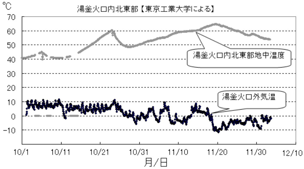
図6 草津白根山 湯釜火口内北東部の噴気地帯 地中温度と外気温 (2008年10月1日~2008年12月3日)
