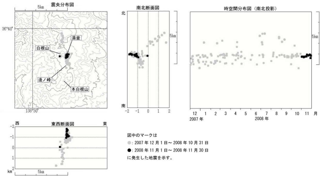
図7 草津白根山 震源分布図(2007年12月1日~2008年11月30日)
