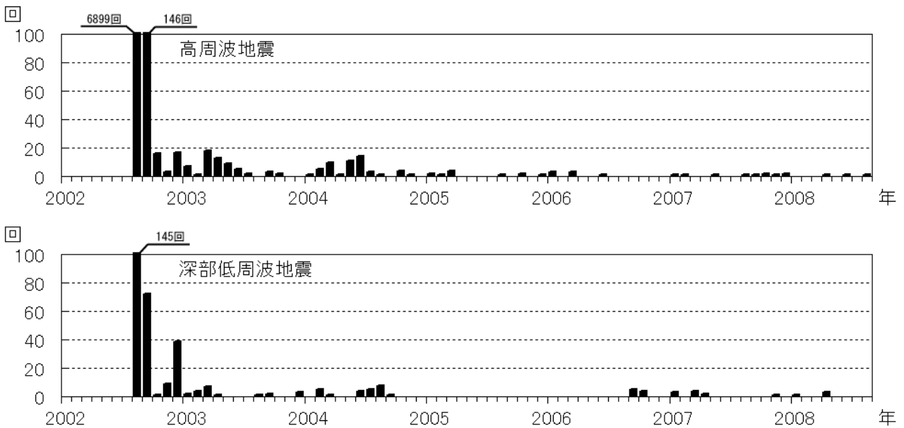
図 1 八丈島 月別地震回数(2002 年 1 月～2008 年 8 月)
