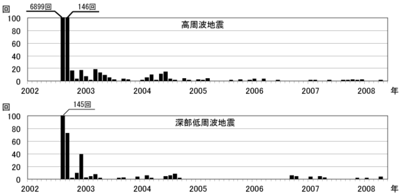
図 1 八丈島 月別地震回数(2002 年 1 月～2008 年 5 月)
