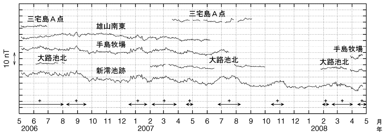
図4 三宅島 全磁力連続観測による全磁力値の変化 (2006年5月～2008年4月30日) ←→で示した期間の全磁力値は三宅島周辺の海流の影響を受けていると推測されます。 nT (ナノテスラ) は磁場の強さを表す単位です。
