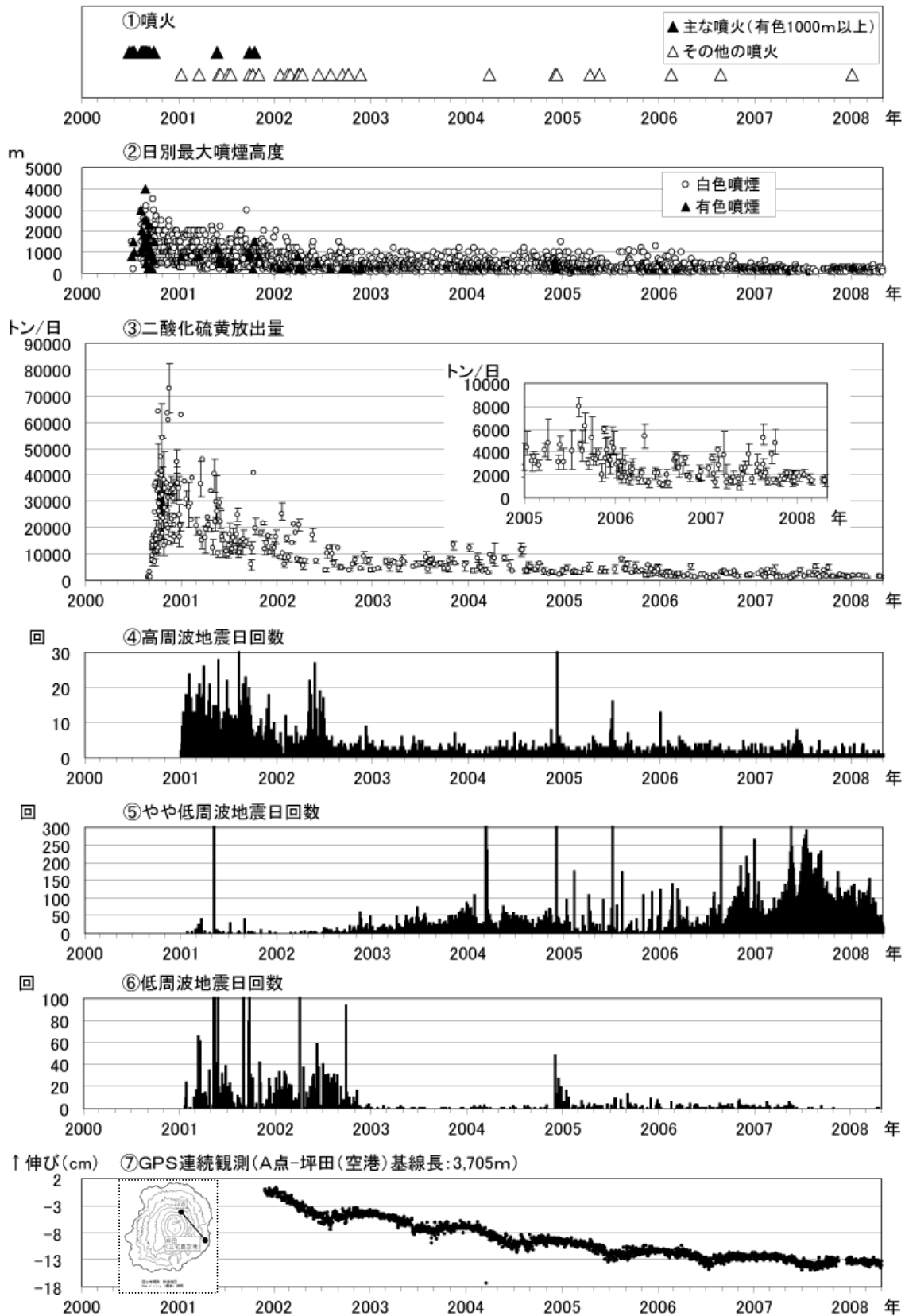
図2 三宅島 最近の火山活動の推移 (2000年1月~2008年4月)
