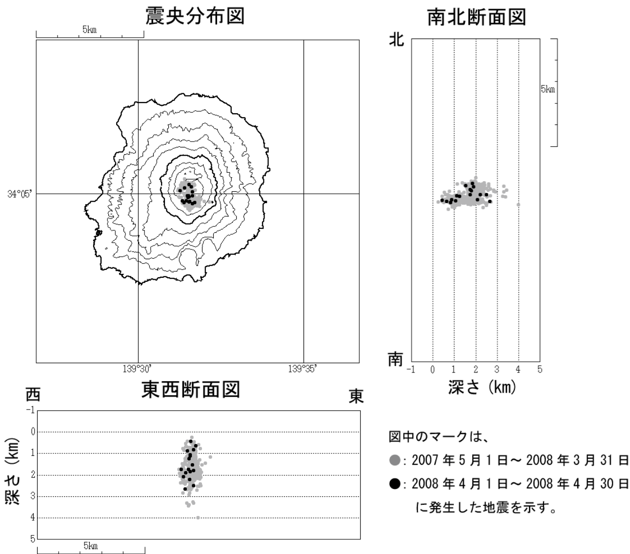
図3※ 三宅島 火山性地震の震源分布 (2007年5月1日～2008年4月30日)
