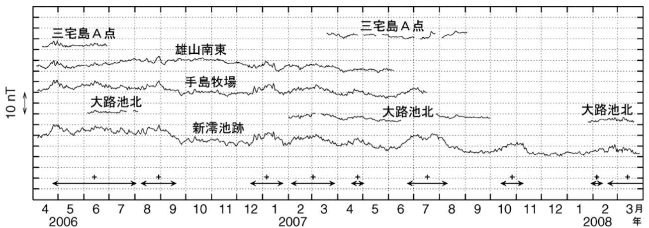
図4 三宅島 全磁力連続観測による全磁力値の変化 (2006年4月～2008年3月31日) ←→で示した期間の全磁力値は三宅島周辺の海流の影響を受けていると推測されます。 nT (ナノテスラ) は磁場の強さを表す単位です。
