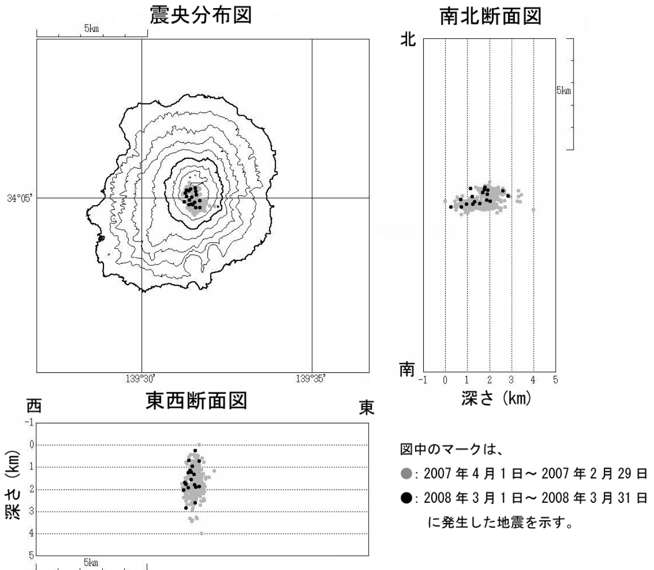
図3※ 三宅島 火山性地震の震源分布 (2007年4月1日～2008年3月31日)
