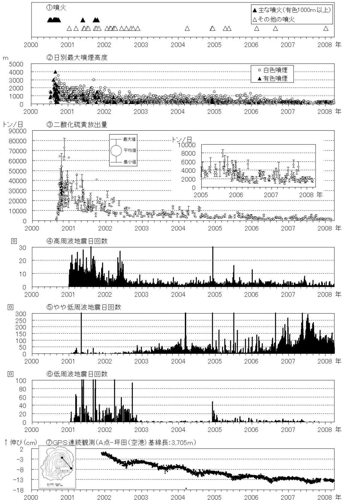
図 2 三宅島 最近の火山活動の推移 (2000 年 1 月～2008 年 3 月)
