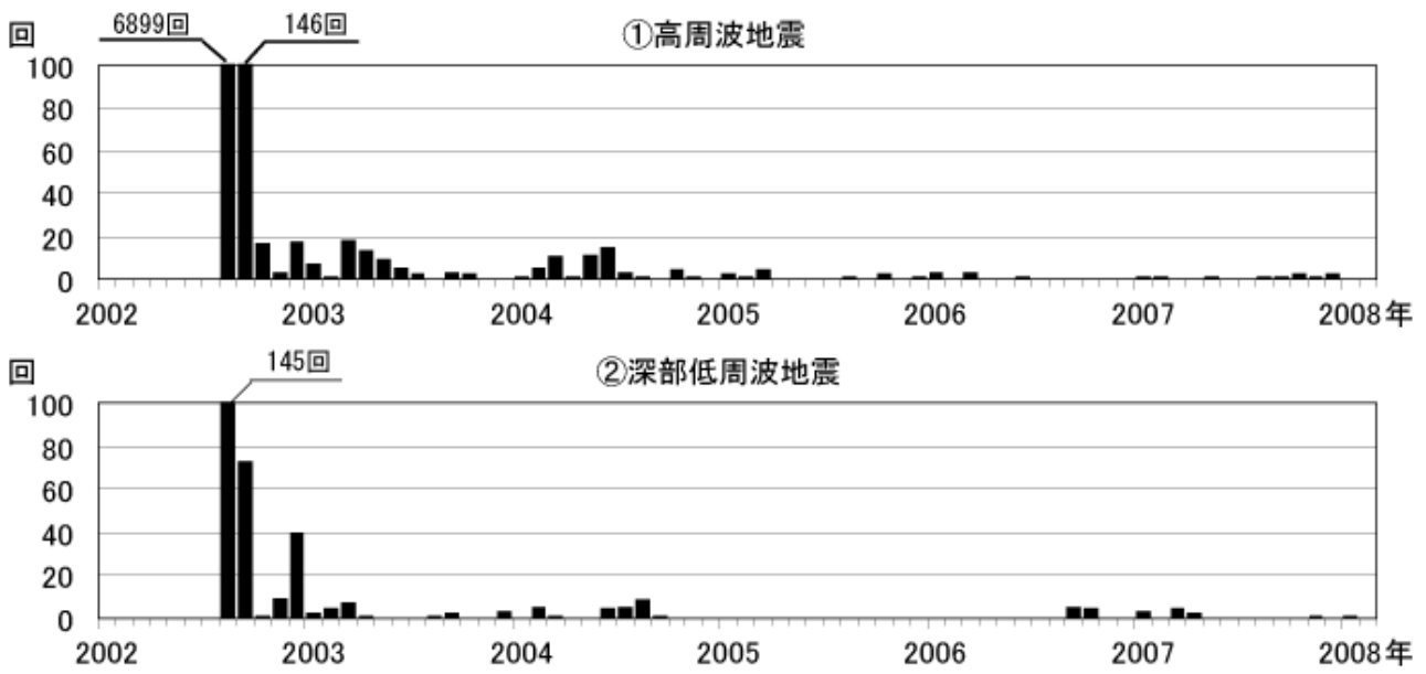
図 1 八丈島 月別地震回数(2002 年 1 月～2008 年 2 月)
