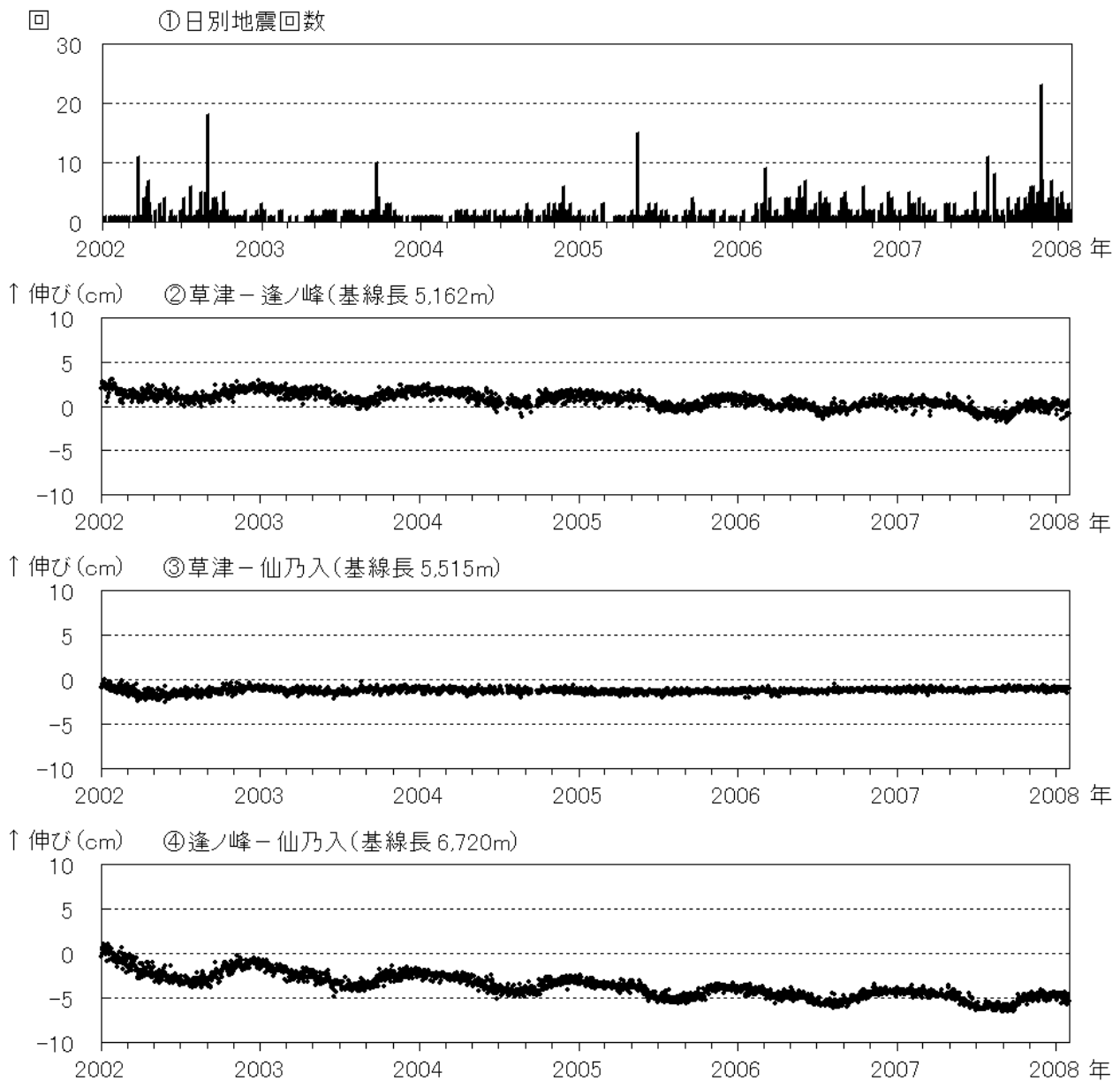
図4 草津白根山 最近の火山活動の推移(2002年1月~2008年1月)
