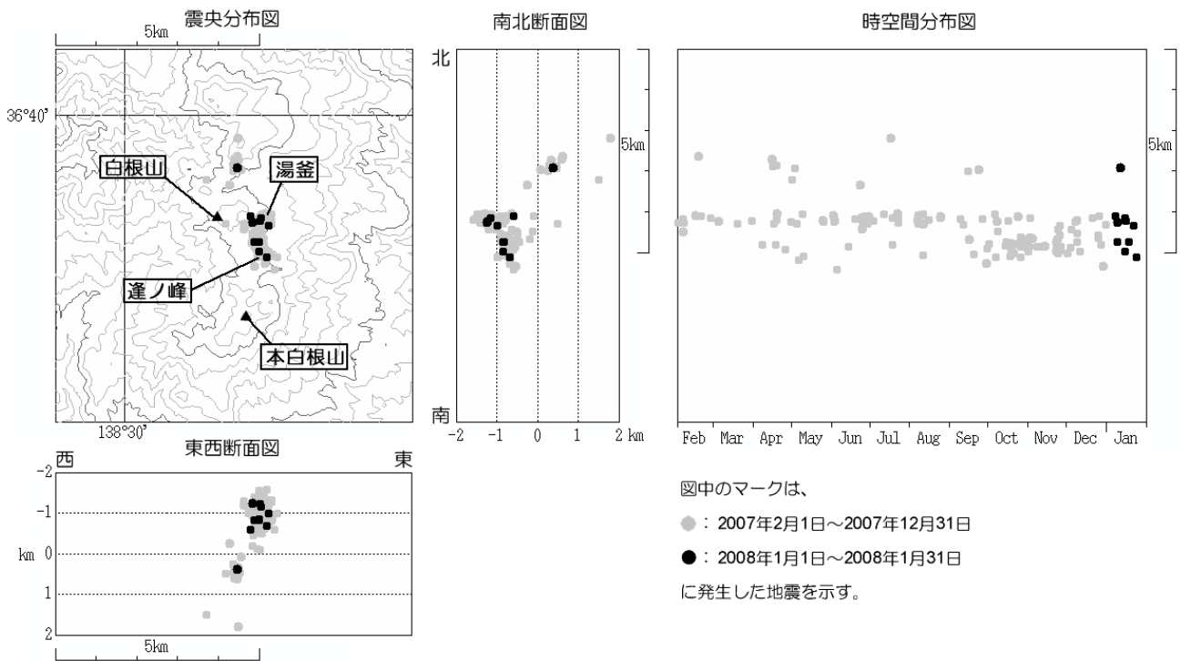
図3 草津白根山 火山性地震の震源分布(2007年2月1日～2008年1月31日)
