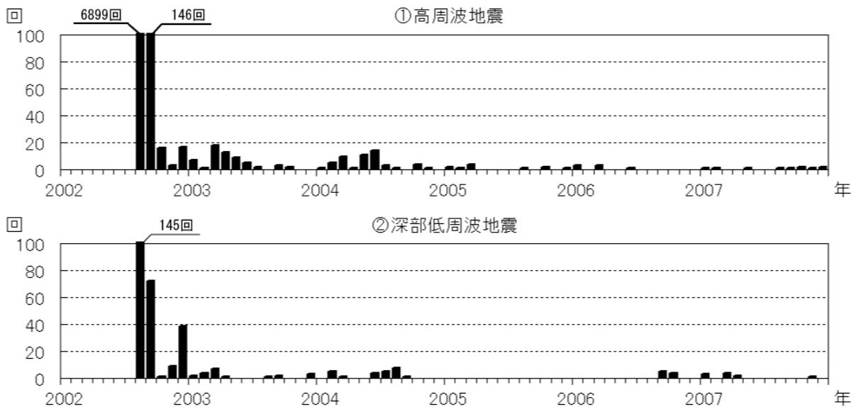
図 1※ 八丈島 月別地震回数(2002 年 1 月～2007 年 12 月)
