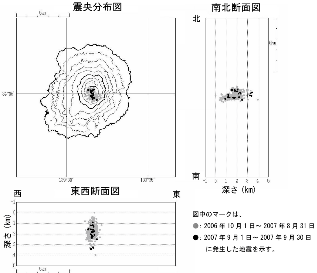
図4※ 三宅島 火山性地震の震源分布 (2006年10月1日～2007年9月30日)
