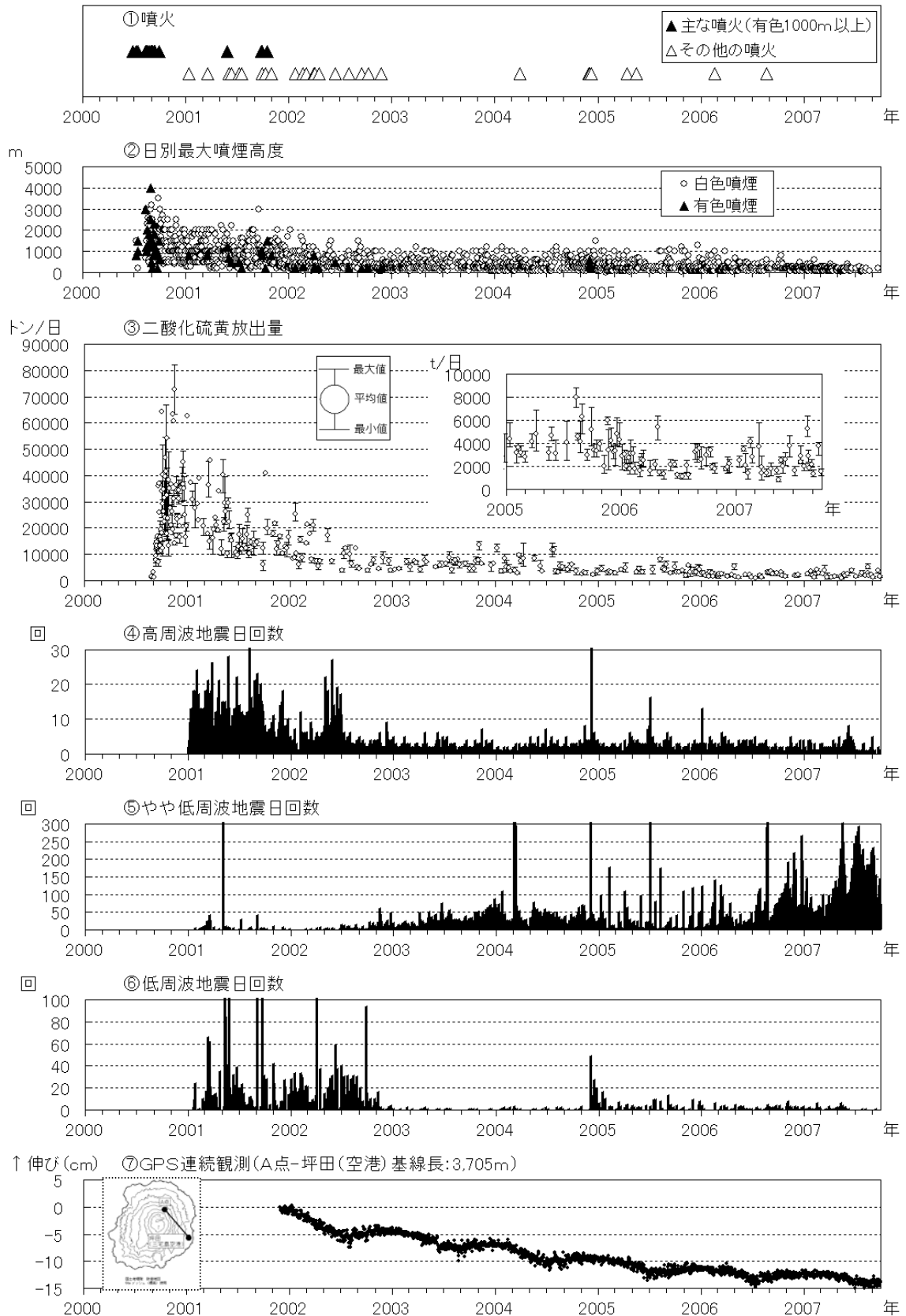
図 3 三宅島 最近の火山活動の推移（2000 年 1 月～2007 年 9 月）
