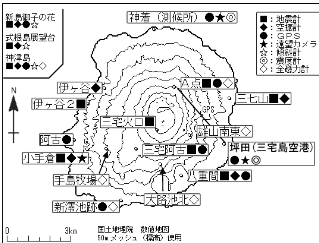
図 2 三宅島 気象庁の観測点配置図（小さな白丸は観測点位置を示しています）
