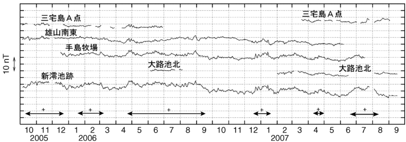
図5 三宅島 全磁力連続観測による全磁力値の変化 (2005年10月1日～2007年9月20日) ←→で示した期間の全磁力値は三宅島周辺の海流の影響を受けていると推測されます。 nT (ナノテスラ) は磁場の強さを表す単位です。
