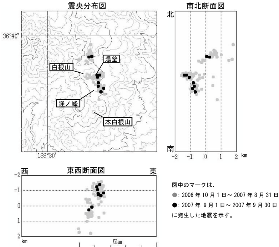
図 2 ※ 草津白根山 火山性地震の震源分布 (2006 年 10 月 1 日～2007 年 9 月 30 日)
