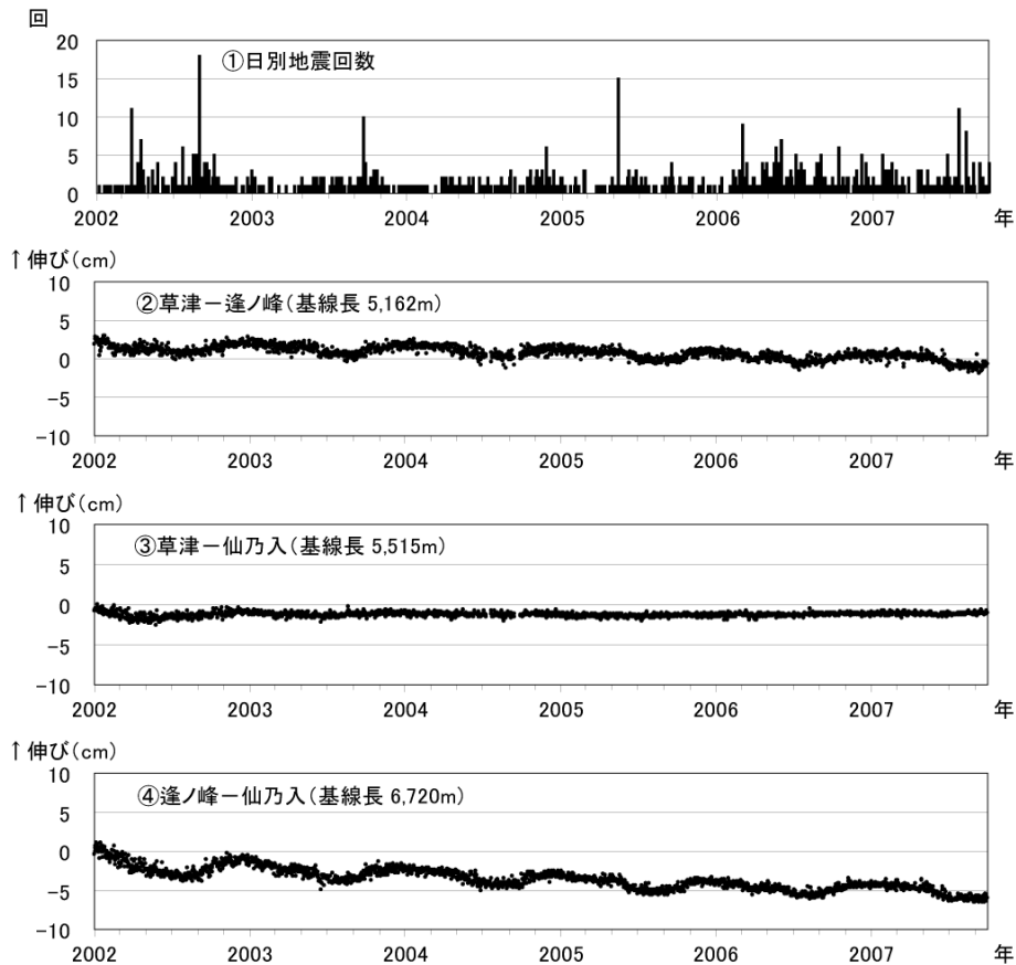
図 3 草津白根山 最近の火山活動の推移 (2002 年 1 月～2007 年 9 月)
