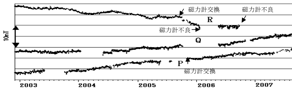
図 6 草津白根山 全磁力連続観測の結果（2002 年 12 月～2007 年 8 月） nT（ナノテスラ）は磁場の強さを表す単位。
