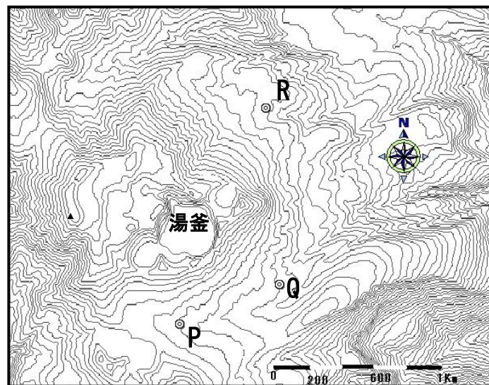
図 5 草津白根山の全磁力連続観測点配置図
