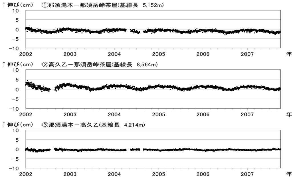
図 3 那須岳 GPS 連続観測による基線長変化 (2002 年 1 月～2007 年 9 月) 基線長変化にみられる冬季の伸びと夏季の縮みの傾向は季節変動による変化です。 ①～③は図 4 の GPS 基線①～③に対応しています。
