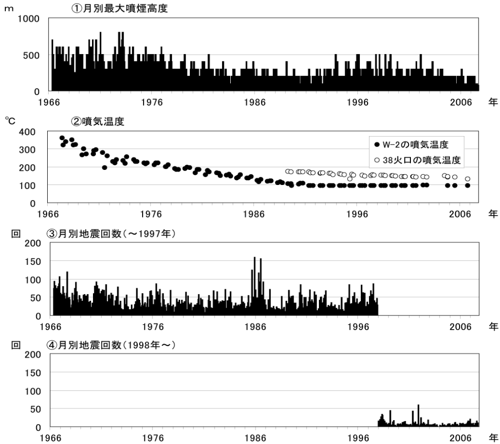
図 2 ※ 那須岳 最近の火山活動の推移 (1966 年 1 月～2007 年 9 月) ①定時観測 (09 時・15 時) による茶臼岳の月別最大噴煙高度 ②噴気温度 (W-2 及び 38 火口はいずれも茶臼岳西側斜面の温度観測定点) ③那須岳周辺も含めた地震の月別回数 ④那須岳山体付近に発生した地震の月別回数
