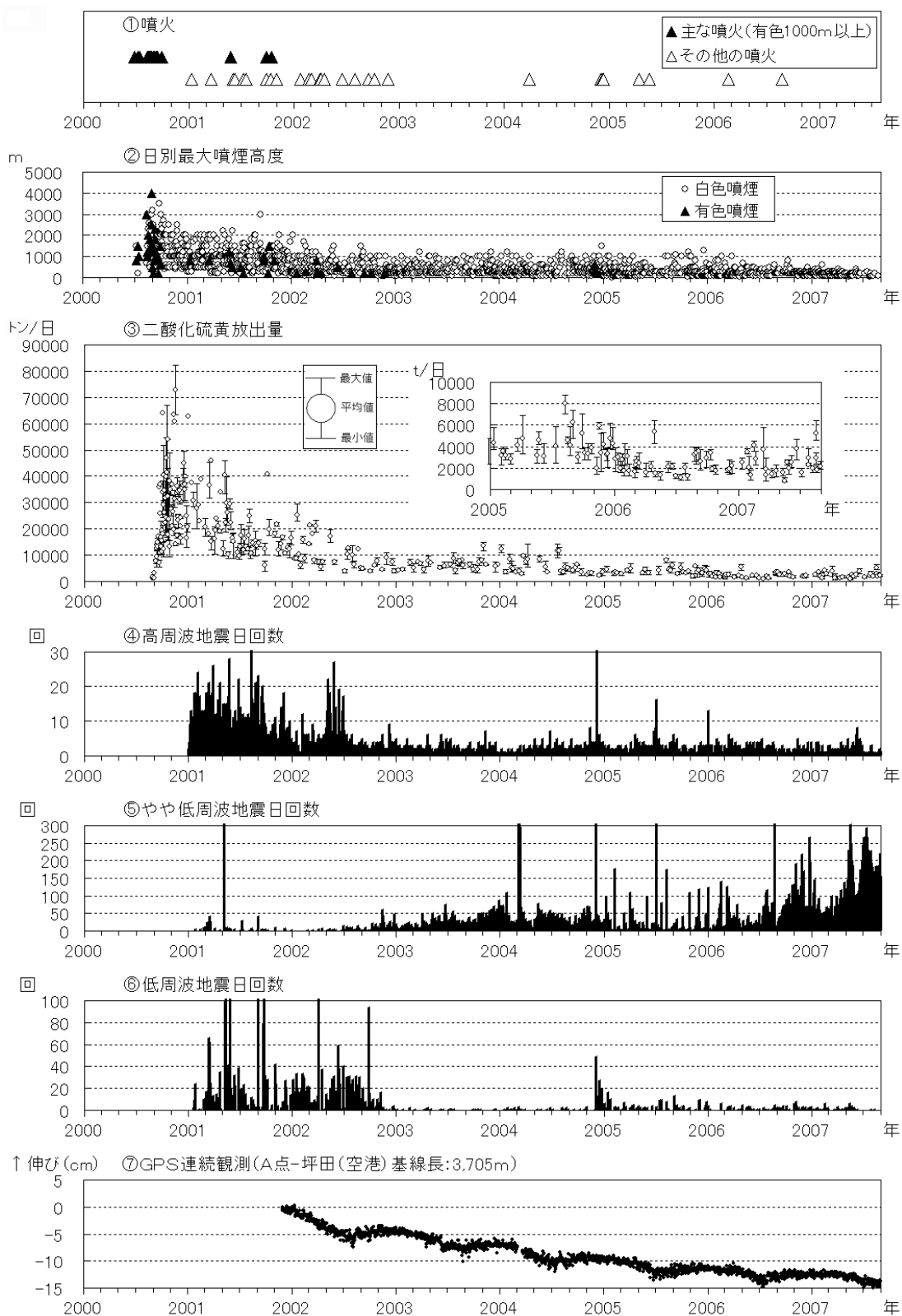
図 2 三宅島 最近の火山活動の推移（2000 年 1 月～2007 年 8 月）
