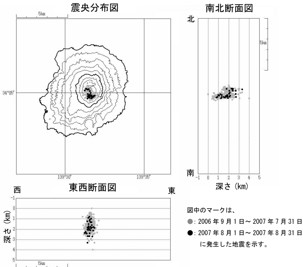
図3 三宅島 火山性地震の震源分布（2006年9月1日～2007年8月31日）
