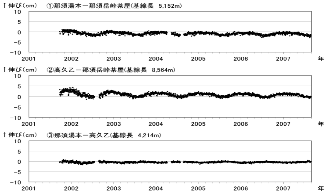
図3 那須岳 GPS連続観測による基線長変化(2002年1月~2007年8月) 基線長変化にみられる冬季の伸びと夏季の縮みの傾向は季節変動による変化です。 ~ は図4のGPS基線 ~ に対応しています。
