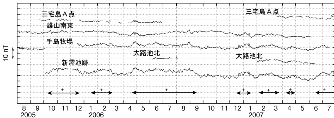
図4 三宅島 全磁力連続観測による全磁力値の変化（2005年6月1日～2007年7月31日） ←→で示した期間の全磁力値は三宅島周辺の海流の影響を受けていると推測されます。 nT（ナノテスラ）は磁場の強さを表す単位です。
