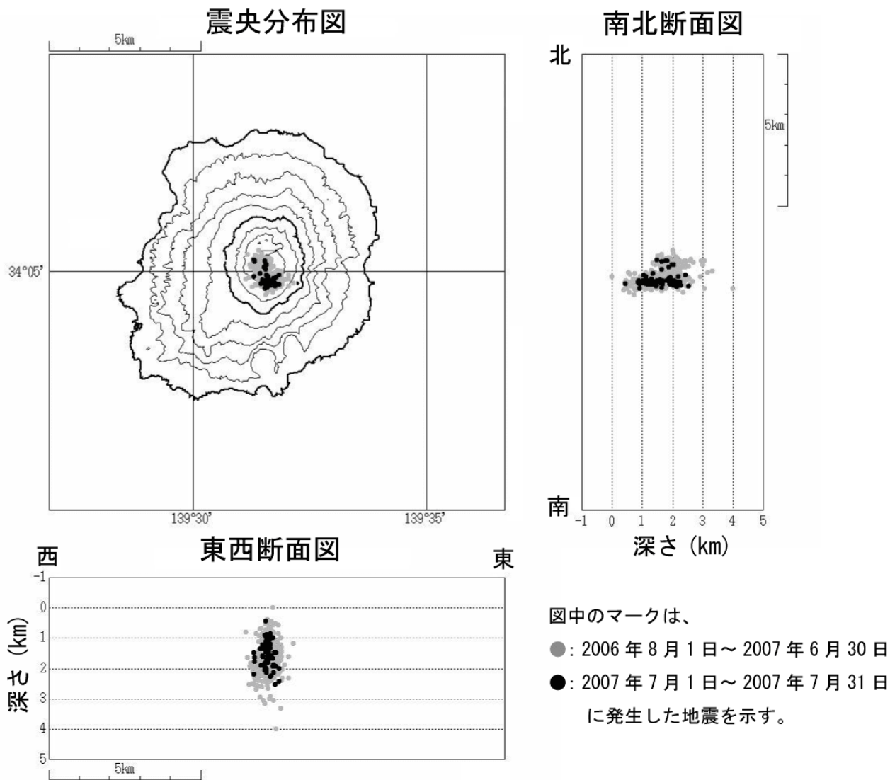
図3 三宅島 火山性地震の震源分布（2006年8月1日～2007年7月31日）
