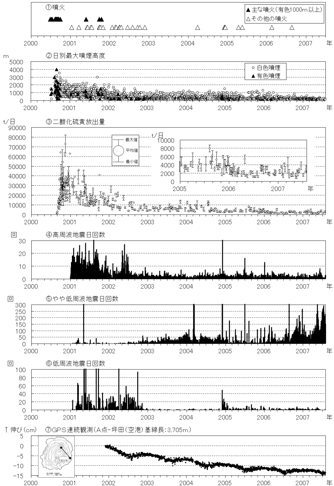
図2 三宅島 最近の火山活動の推移（2000年1月～2007年7月）
