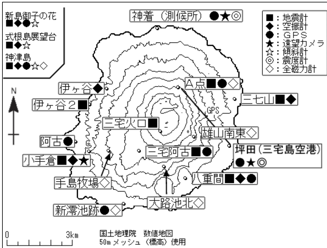
図 7 三宅島 気象庁の観測点配置図（小さな白丸は観測点位置を示しています） GPS 基線（A 点 - 坪田）は図 3 の に対応しています。
