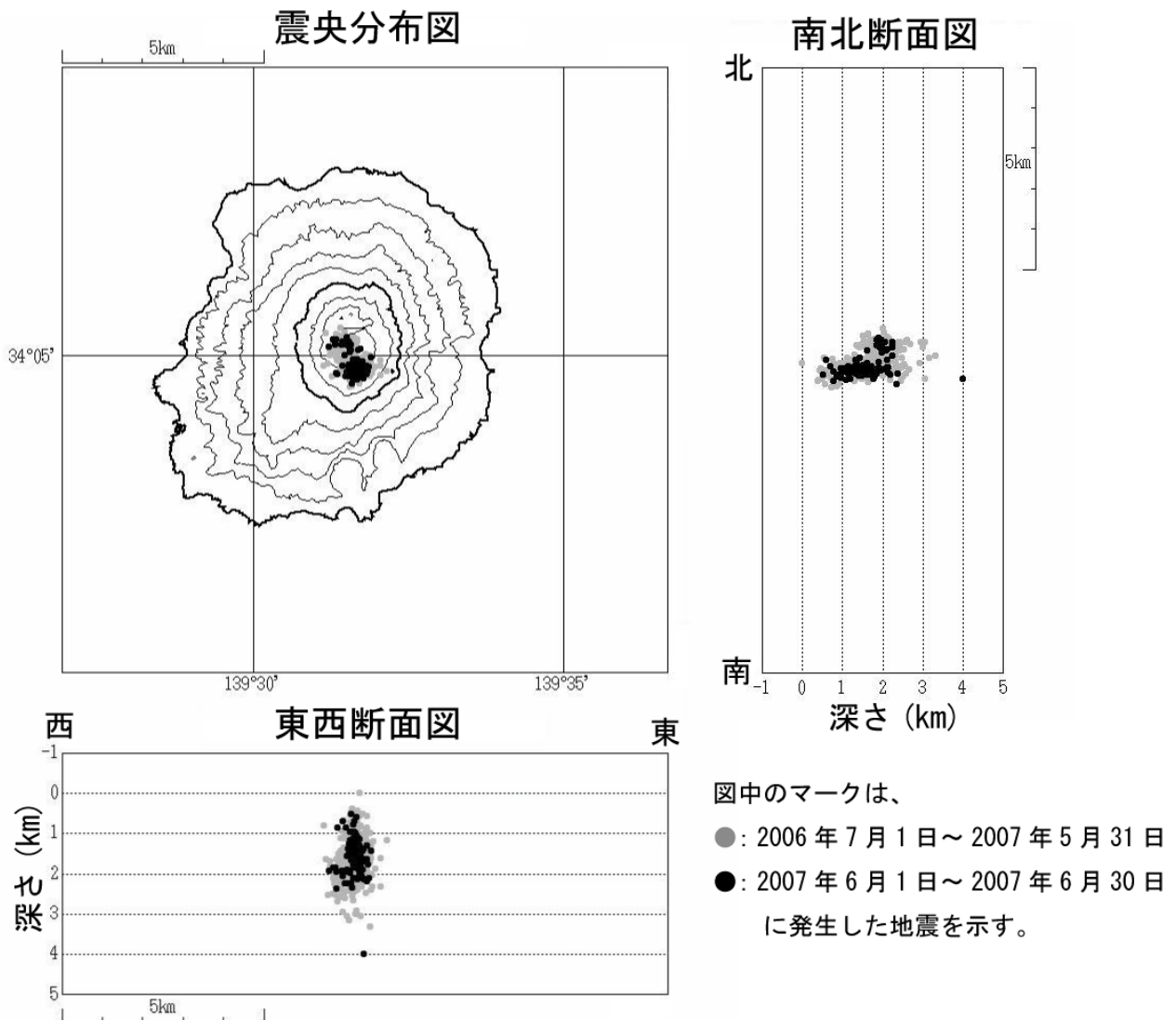
図4 三宅島 火山性地震の震源分布（2006年7月1日～2007年6月30日）
