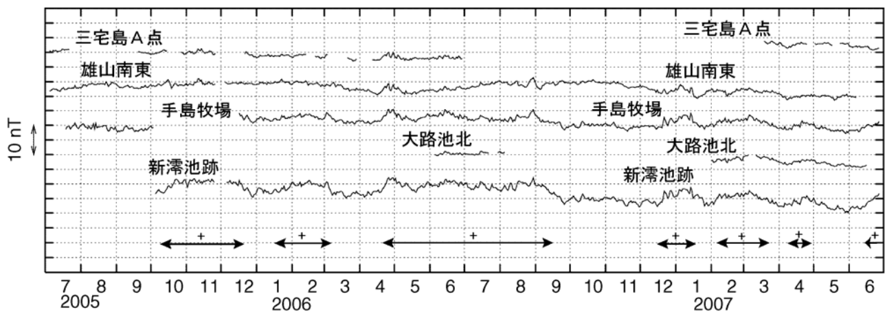
図5 三宅島 全磁力連続観測による全磁力値の変化（2005年6月1日～2007年6月30日） ←→で示した期間の全磁力値は三宅島周辺の海流の影響を受けていると推測されます。 nT（ナノテスラ）は磁場の強さを表す単位です。
