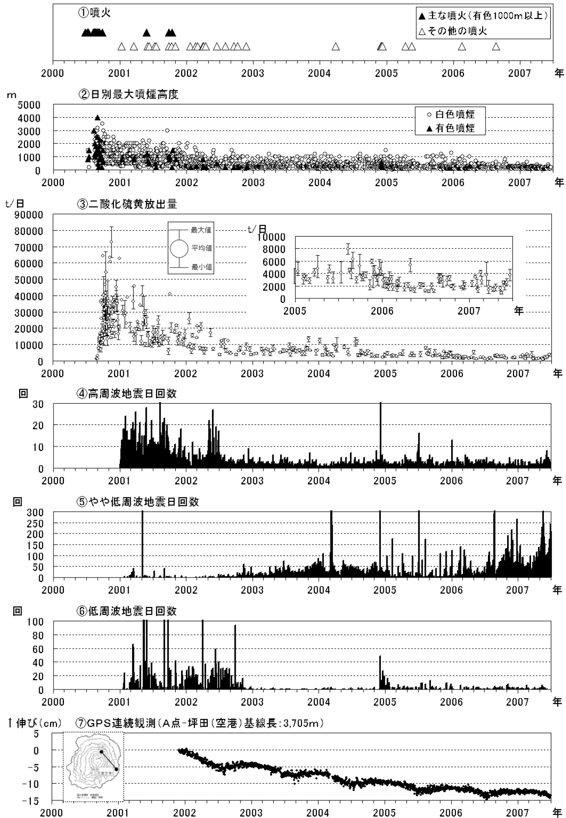
図3 三宅島 最近の火山活動の推移（2000年1月～2007年6月）
