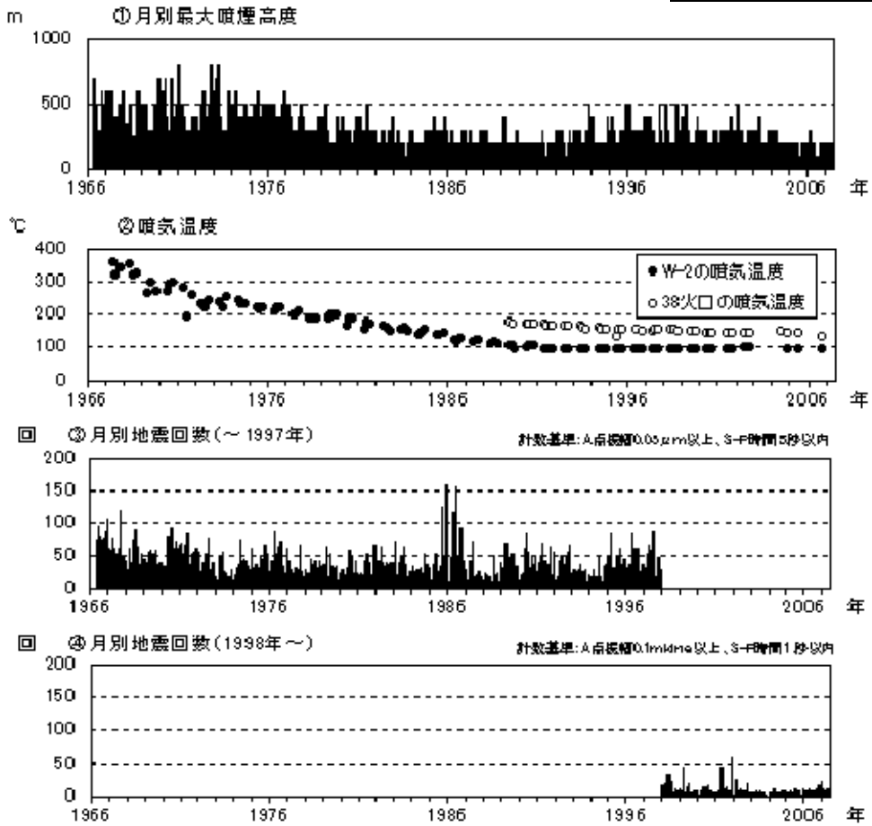
図2 那須岳 最近の火山活動の推移(1966年1月~2007年6月) 定時観測(09時・15時)による茶臼岳の月別最大噴煙高度 噴気温度(W-2及び38火口はいずれも茶臼岳西側斜面の温度観測定点) 那須岳周辺も含めた地震の月別回数 那須岳山体付近に発生した地震の月別回数
