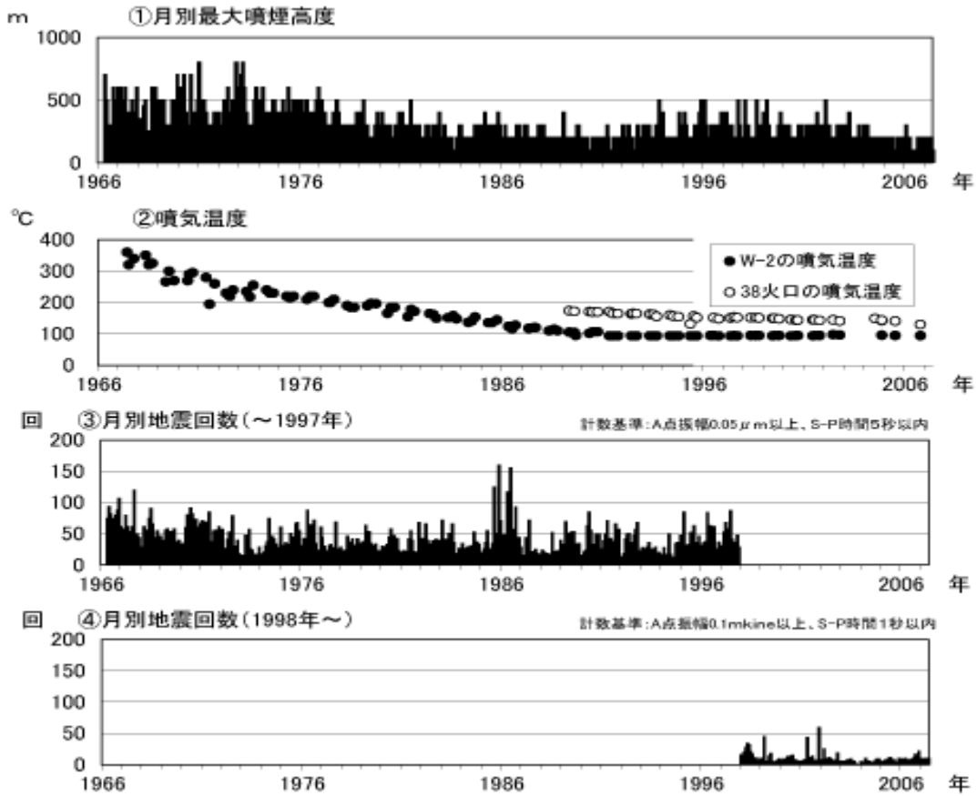
図 2※ 那須岳 最近の火山活動の推移 (1966 年 1 月～2007 年 5 月) ① 定時観測 (09 時・15 時) による茶臼岳の月別最大噴煙高度 ② 噴気温度 (W-2 及び 38 火口はいずれも茶臼岳西側斜面の温度観測定点) ③ 那須岳周辺も含めた地震の月別回数 ④ 那須岳山体付近に発生した地震の月別回数
