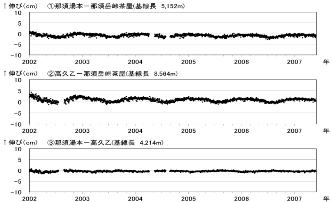
図 3 那須岳 GPS 連続観測による基線長変化 (2002 年 1 月～2007 年 5 月) 基線長変化にみられる冬季の伸びと夏季の縮みの傾向は季節変動による変化です。 ①～③は図 4 の GPS 基線①～③に対応しています。
