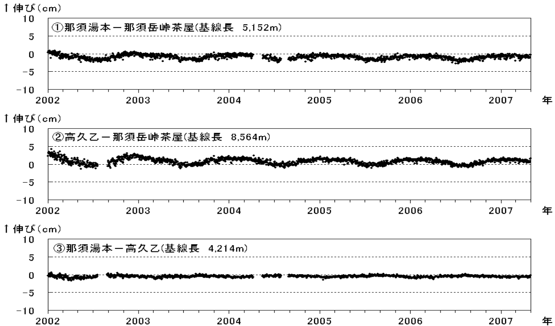
図 3 那須岳 GPS 連続観測による基線長変化 (2002 年 1 月~2007 年 4 月) 基線長変化にみられる冬季の伸びと夏季の縮みの傾向は季節変動による変化です。 ①~③は図 4 の GPS 基線①~③に対応しています。
