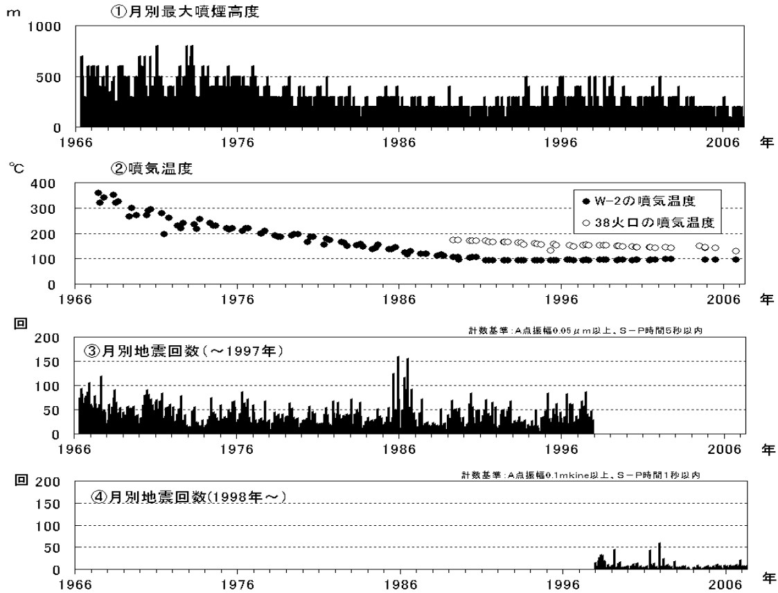
図 2※ 那須岳 最近の火山活動の推移 (1966 年 1 月~2007 年 4 月) ① 定時観測 (09 時・15 時) による茶臼岳の月別最大噴煙高度 ② 噴気温度 (W-2 及び 38 火口はいずれも茶臼岳西側斜面の温度観測定点) ③ 那須岳周辺も含めた地震の月別回数 ④ 那須岳山体付近に発生した地震の月別回数
