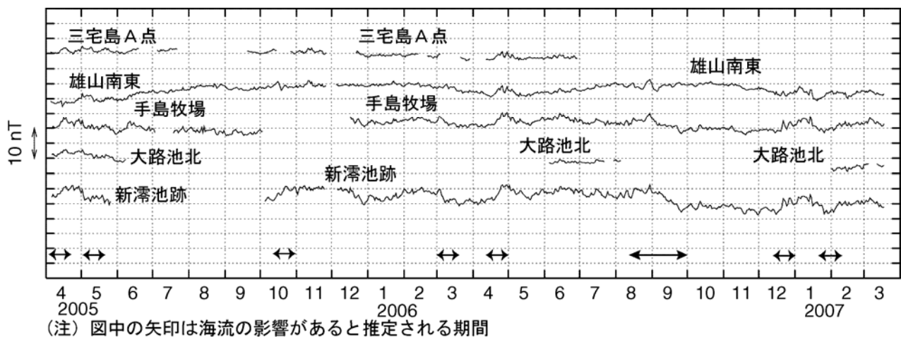
図5 三宅島 全磁力連続観測による全磁力値の変化 (2004年12月1日～2007年3月31日) ←→で示した期間の全磁力値は三宅島周辺の海流の影響を受けていると推定されます。 nT (ナノテスラ) は磁場の強さを表す単位です。
