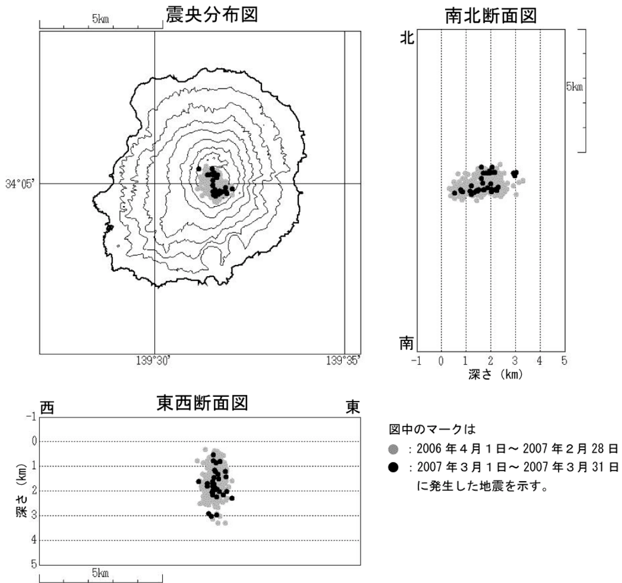
図4※ 三宅島 火山性地震の震源分布 (2006年4月1日～2007年3月31日)
