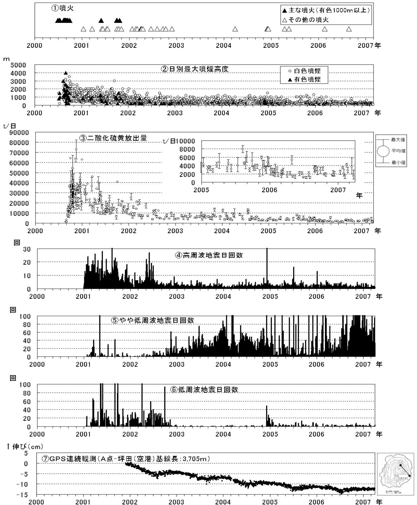
図3 三宅島 最近の火山活動の推移（2000年1月～2007年3月）
